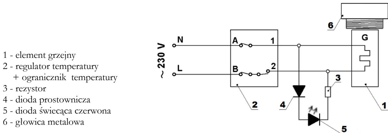
Rys. 3 Schemat elektryczny podgrzewacza z grzałką elektryczną 1- fazową
