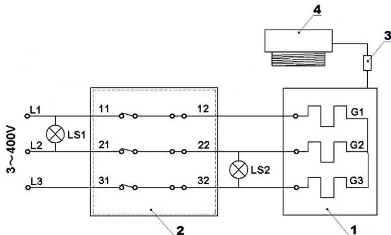
Rys. 5 Schemat elektryczny podgrzewacza z grzałką elektryczną 3- fazową
