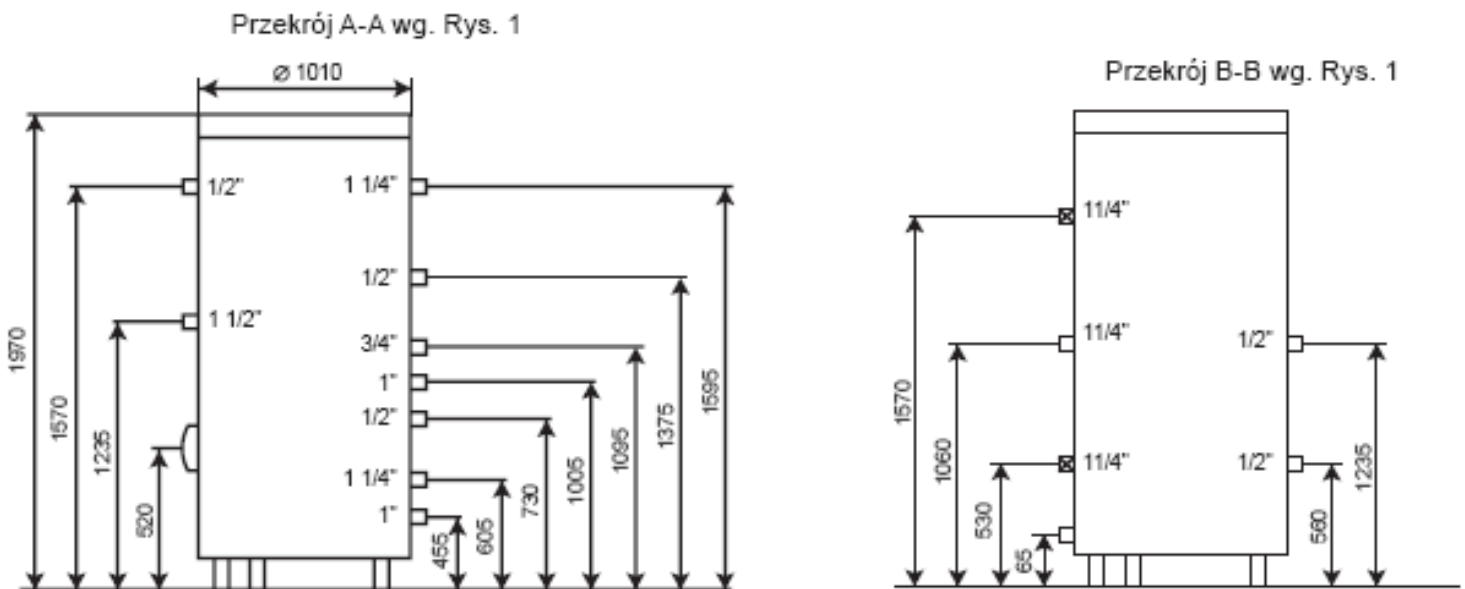
Rys. 2 Wymiary podgrzewacza
