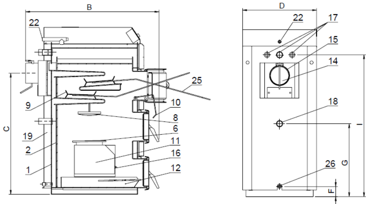
Rys. 1. Konstrukcja i wymiary kotłów EKO-KWP ns
