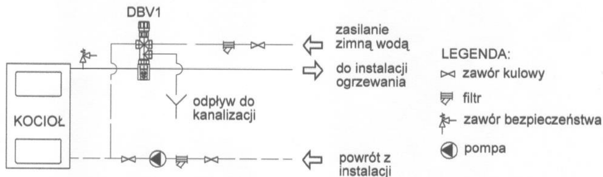
Rys.5 Schemat instalacji z dwudrogowym zaworem bezpieczeństwa DBV1.
