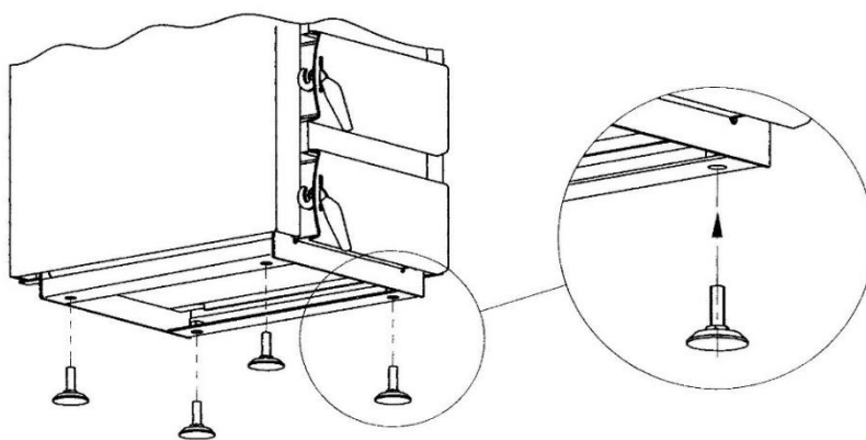
Rys. 4. Pозиomowanie kotła
