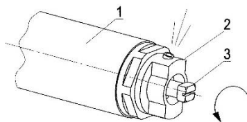
Rys.9. Odpowietrznik: 1 - rura odpowietrznika, 2 - odpowietrznik, 3 - wkręt.
