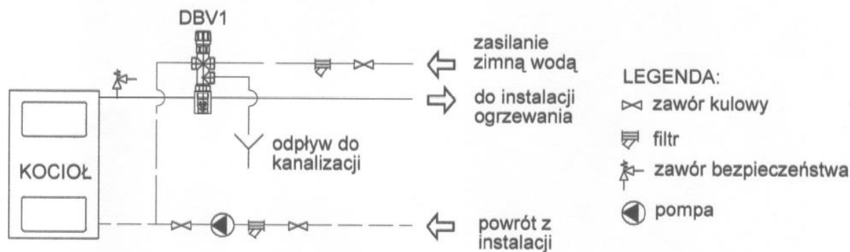
Rys.9 Schemat instalacji z dwudrogowym zaworem bezpieczeństwa DBV1.
