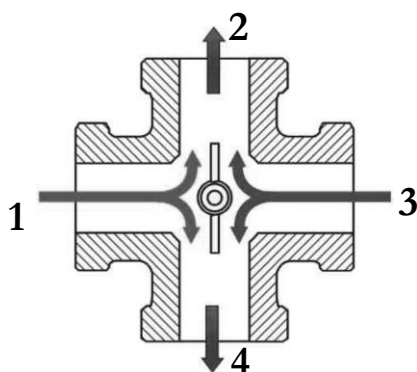
Rys. 11. Czterodrogowy zawór mieszający
