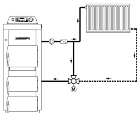
Rys.12a. Przykład montażu zaworu mieszającego w instalacji z regulacją ilościową (zapewnia ochronę kotła przed „zimnym” powrotem czynnika grzewczego).
