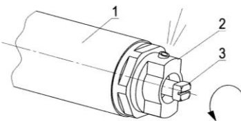
Rys.14. Odpowietrznik: 1 - rura odpowietrznika, 2 - odpowietrznik, 3 - wkręt.
