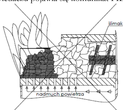
Rys.18 Zbyt duża podaż paliwa; spychanie niedopalonego paliwa z retorty
