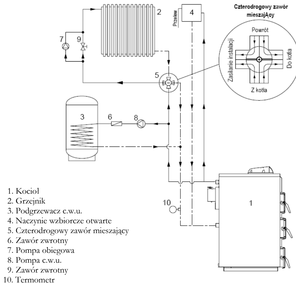
Rys. 13. Przykładowy schemat podłączenia kotła do systemu grzewczego c.o. i c.w.u. z wykorzystaniem czterodrogowego zaworu mieszającego.
