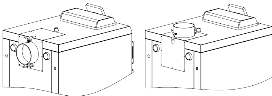
Rys.2 Możliwości montażu czopucha
