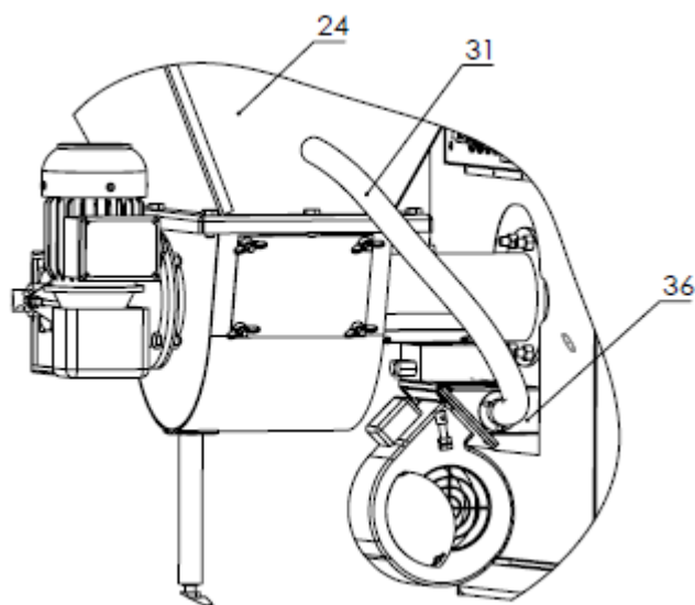
Rys. 6 Wyrównanie ciśnienia powietrza w zasobniku paliwa i w komorze mieszacza
