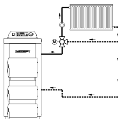
Rys.12b. Przykład montażu zaworu mieszającego w instalacji z regulacją jakościową (nie zapewnia ochrony kotła przed „zimnym” powrotem czynnika grzewczego).
