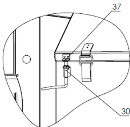
Rys. 4 Czujnik klapy zasobnika
