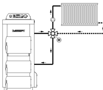
Rys.11a. Przykład montażu zaworu mieszającego czterodrogowego.
