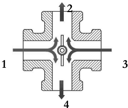
Rys. 10. Czterodrogowy zawór mieszający
