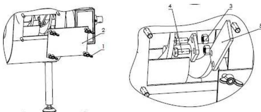
Rys.14. Demontaż zabieraka paliwa
