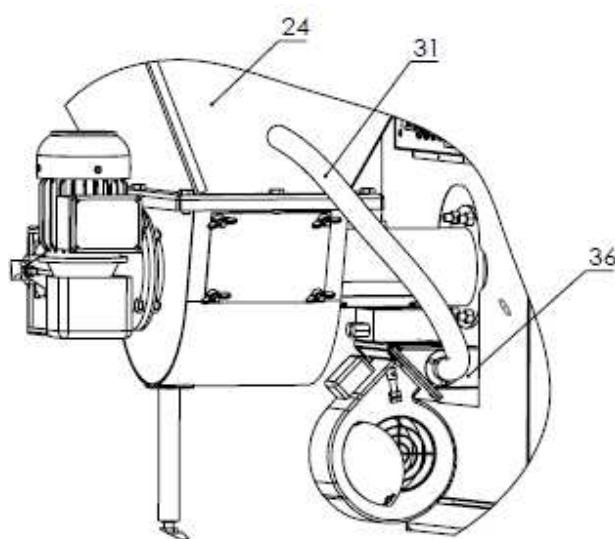
Rys. 5 Wyrównanie ciśnienia powietrza w zasobniku paliwa i w komorze mieszacza
