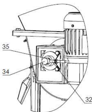
Rys. 4 Czujnik obrotów silnika podajnika
