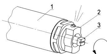
Rys.13. Odpowietrznik: 1 - rura odpowietrznika, 2 - odpowietrznik, 3 - wkręt.
