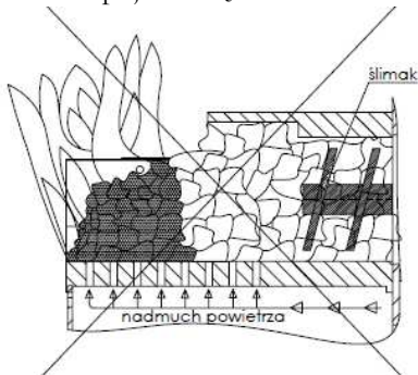
Rys.17 Zbyt duża podaż paliwa; spychanie niedopalonego paliwa z retorty
