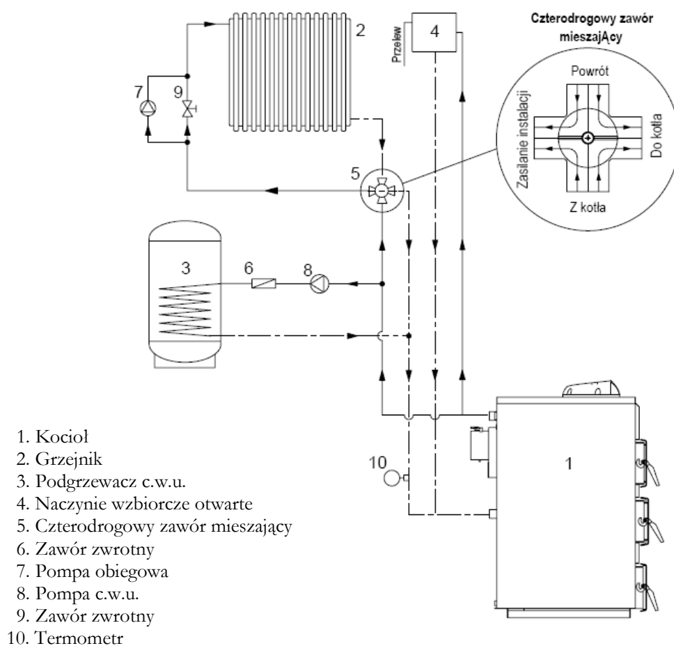
Rys. 12. Przykładowy schemat podłączenia kotła do systemu grzewczego c.o. i c.w.u. z wykorzystaniem czterodrogowego zaworu mieszającego.
