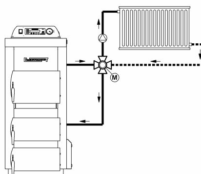
Rys.10a. Przykład montażu zaworu mieszającego czterodrogowego.
