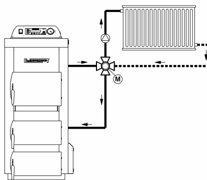
Rys.5a. Przykład montażu zaworu mieszającego czterodrogowego.
