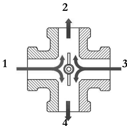
Rys. 5. Czterodrogowy zawór mieszający 1 - zasilanie z kotła 3 - powrót z instalacji 2 - zasilanie instalacji 4 - powrót do kotła
