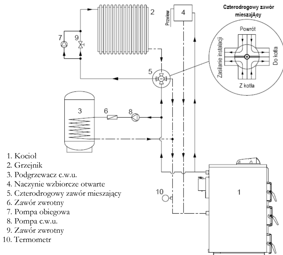
Rys. 7. Przykładowy schemat podłączenia kotła do systemu grzewczego c.o. i c.w.u. z wykorzystaniem czterodrogowego zaworu mieszającego.
