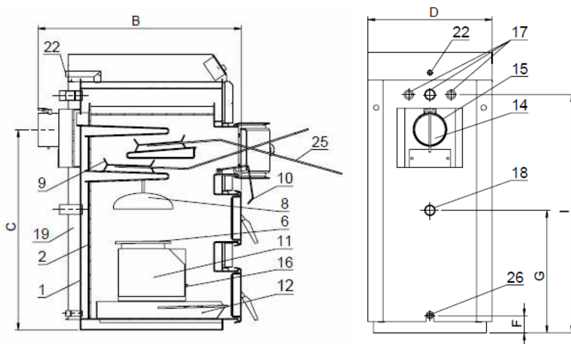
Rys. 1. Konstrukcja i wymiary kotłów EKO-KWP premium
