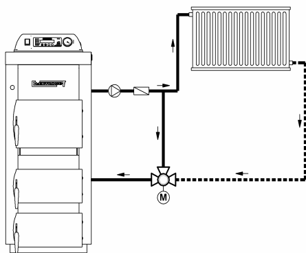
Rys. 6a. Przykład montażu zaworu mieszającego w instalacji z regulacją ilościową (zapewnia ochronę kotła przed „zimnym” powrotem czynnika grzewczego).
