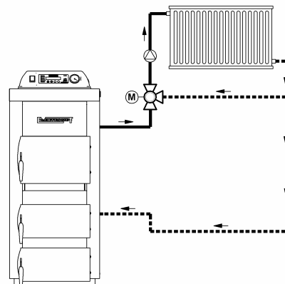
Rys. 6b. Przykład montażu zaworu mieszającego w instalacji z regulacją jakościową (nie zapewnia ochrony kotła przed „zimnym” powrotem czynnika grzewczego).
