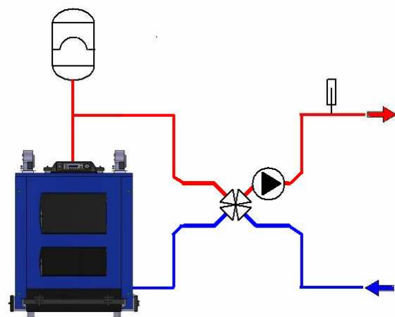
Rys.9 Zawór czterodrogowy
