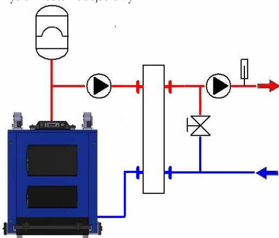
Rys.8 Sprzęgło hydrauliczne
