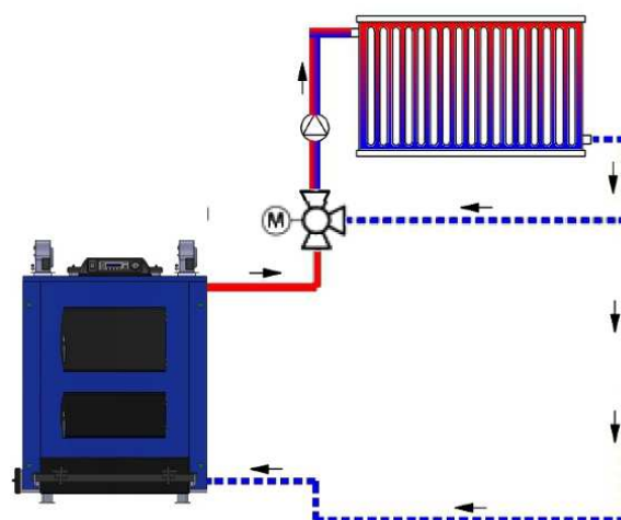
Rys.13 Schemat montażu z regulacją jakościową.
