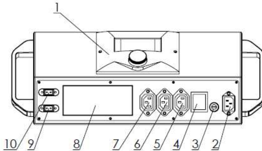
Rys.14 Sterownik EL880 zPID z listwą przyłączeniową.
