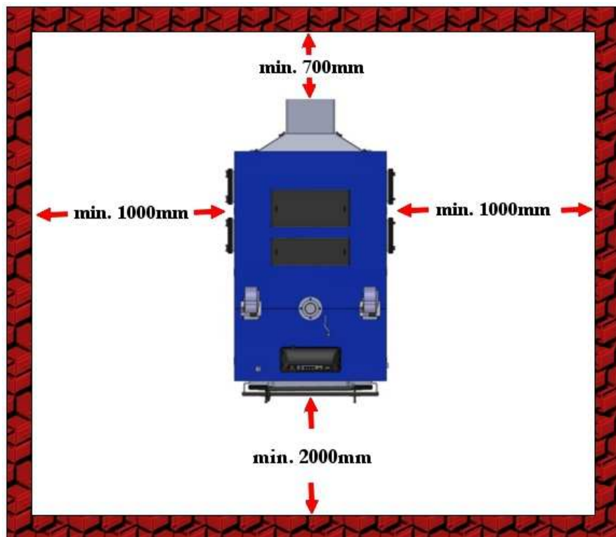
Rys.5 Umieszczenie kotła w kotłowni
