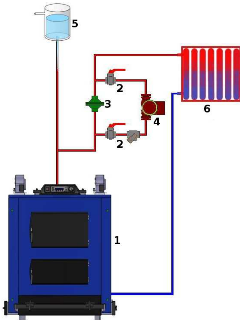
Rys.3 Przykład wykonania obiegu grawitacyjnego
