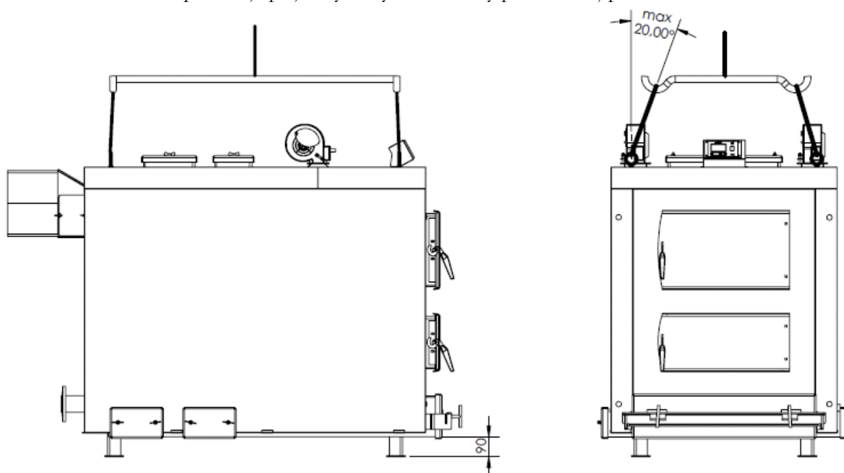
Rys.4 Transport z wykorzystaniem miejsca pod kotłem na łapy transportowe wózka paletowego lub czterech przykręconych przywiesi.
