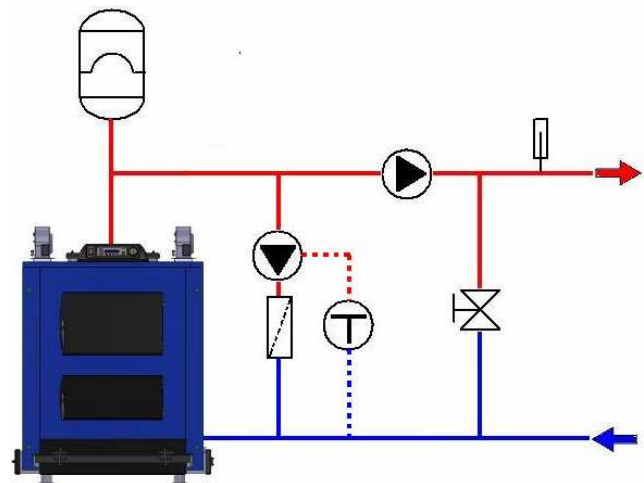
Rys.7 Pompa dozująco mieszająca
