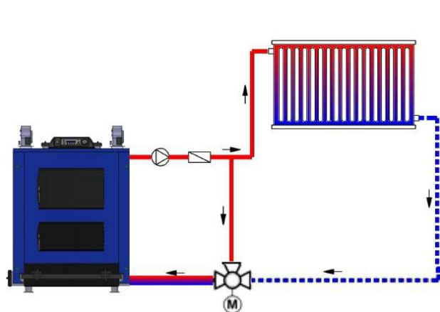
Rys.12 Schemat montażu w konfiguracji ochronnej.
