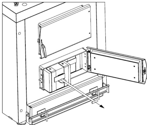
Rys.16 Sposób wyciągnięcia przegrody
