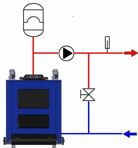
Rys.6 Mostek obejściowy
