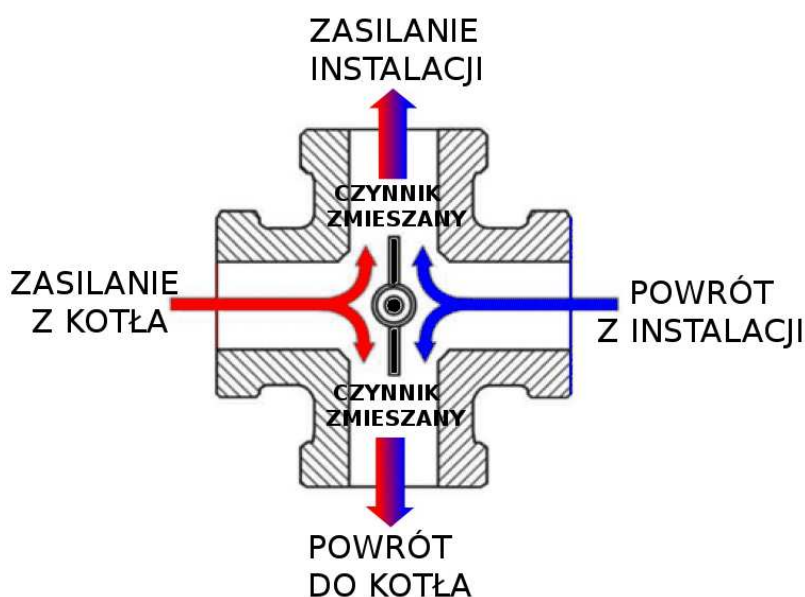
Rys.10 Zawór czterodrogowy.
