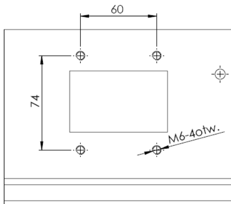
Rys. 3 Rozstaw otworów do zainstalowania wentylatora nadmuchowego do przepustnicy powietrza pierwotnego w drzwiczkach popielnika
