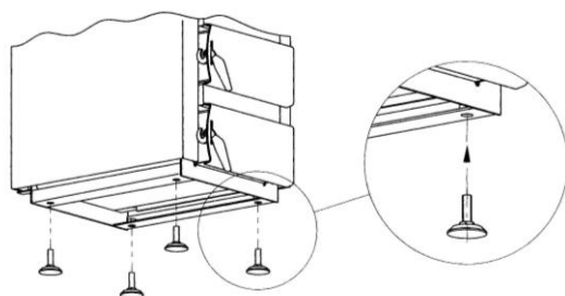
Rys.2 Poziomowanie kotła
