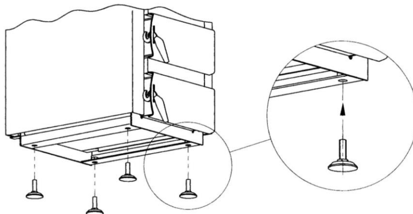
Rys. 5. Pозиomowanie kotła
