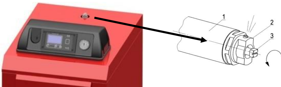
Rys.10. Odpowietrznik: 1 - rura odpowietrznika, 2 - odpowietrznik, 3 - wkręt.
