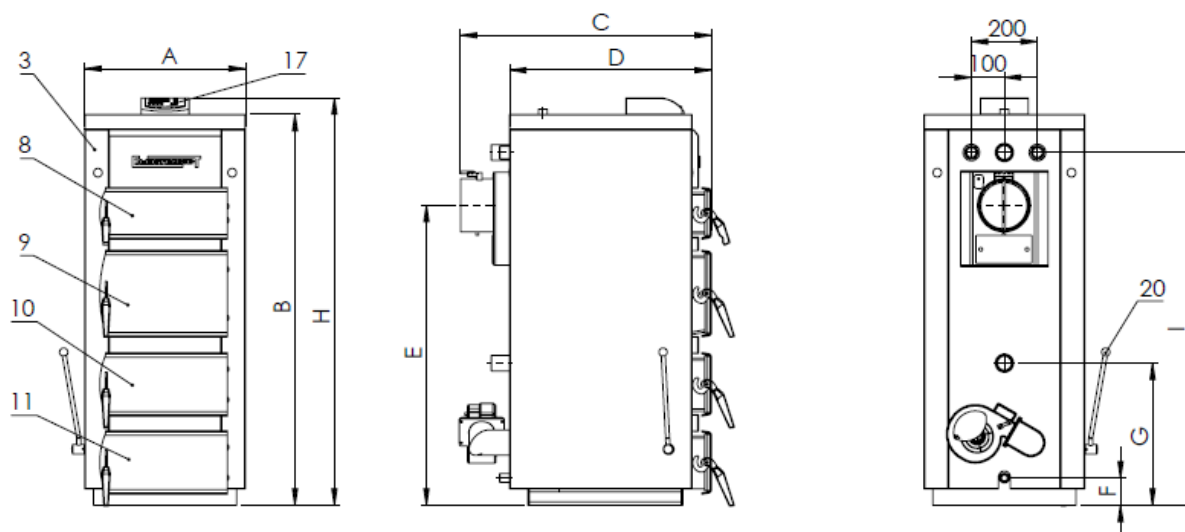
Rys. 2. Wymiary kotłów EKO-KWW STRONG
