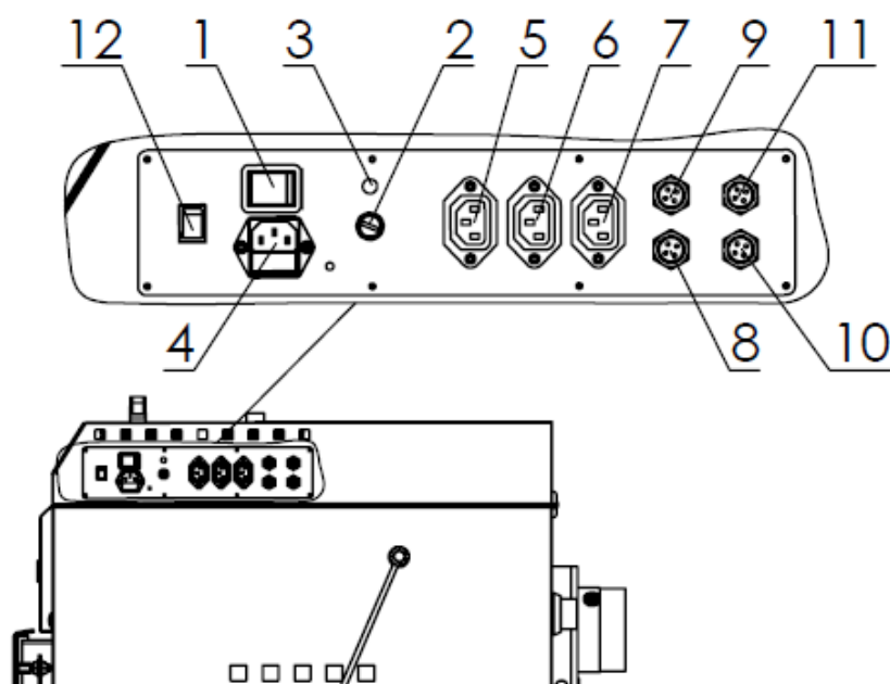
Rys.3 Listwa przyłączeniowa
