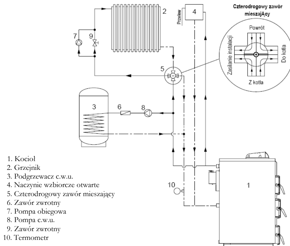
Rys. 9 Przykładowy schemat podłączenia kotła do instalacji c.o. i c.w.u. systemu otwartego z wykorzystaniem czterodrogowego zaworu mieszającego.
