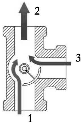
Rys. 8. Trzydrogowy zawór mieszający
