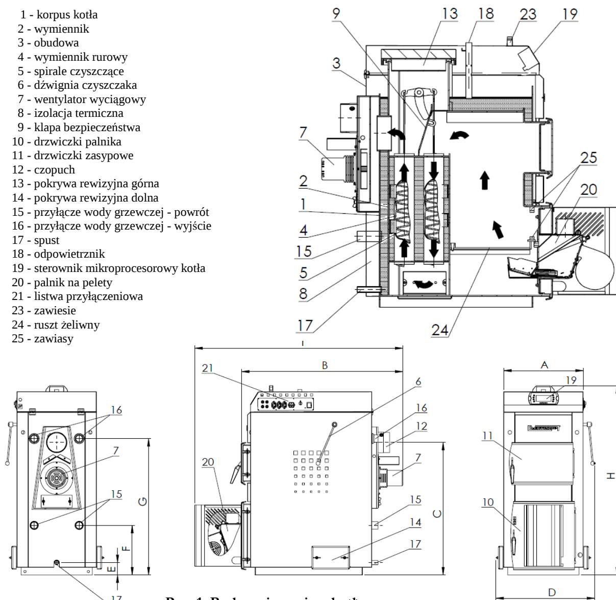
Rys. 1 Budowa i wymiary kotła c.o.
