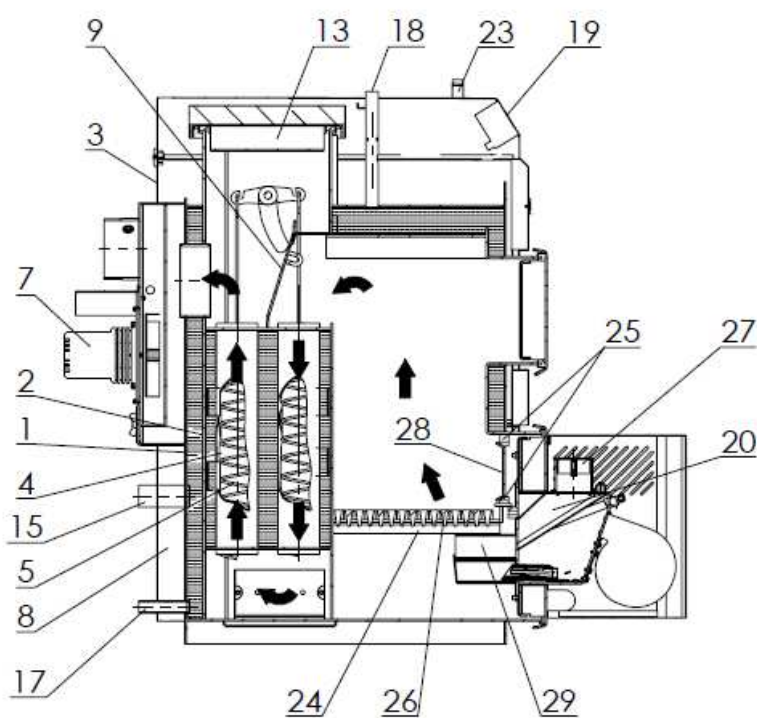
Rys.13 Kocioł EKO-PE dual z rusztem żeliwnym przystosowanym do spalania drewna.
