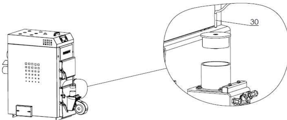
Rys. 11 Zakładanie pokrywy ( poz. 30 - czujnik temperatury podajnika)
