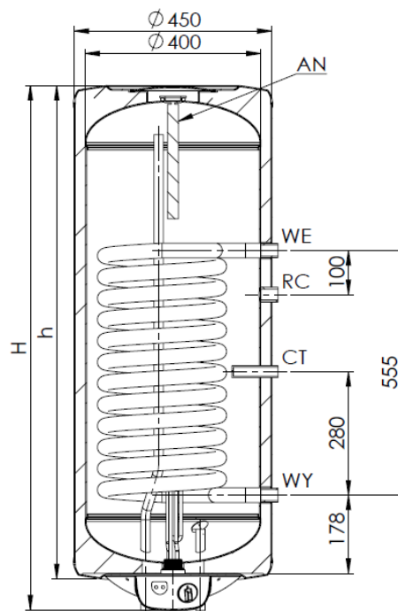
PRZEKRÓJ A-A
