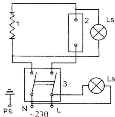
Rys.3 Schemat elektryczny ogrzewacza
