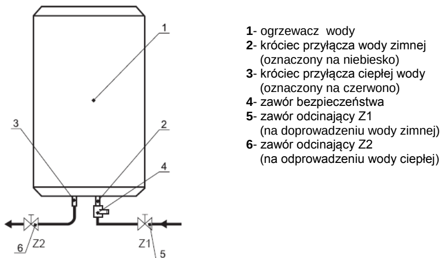
Rys.2 Schemat podłączenia ogrzewacza do sieci wodociągowej
