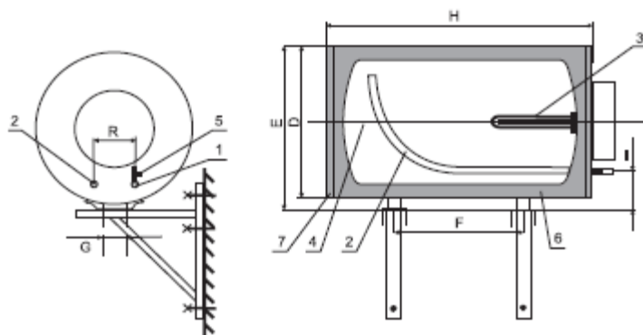
Rys.2 Wymiary gabarytowe ogrzewaczy typu WJ standard 60÷100 – poziome
