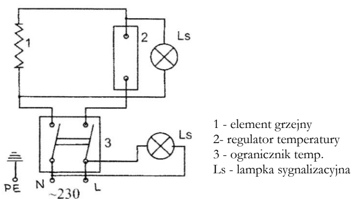
Wersja „VENUS” i „MISTER”.
