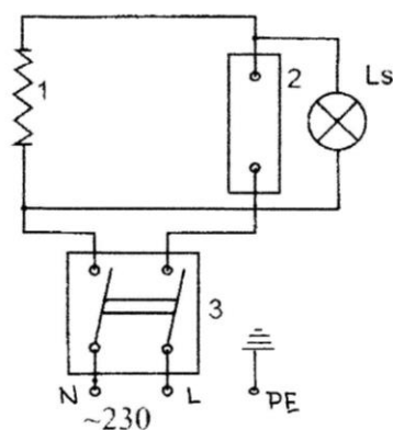
Wersja WJ standard.
