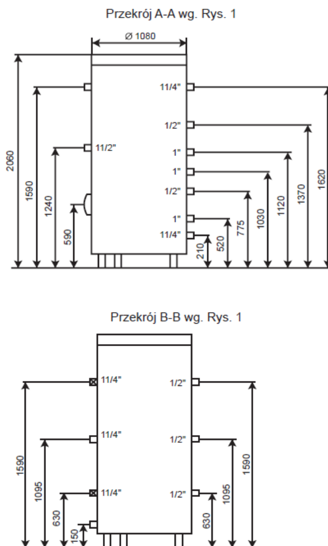
Rys. 2 Wymiary podgrzewacza
