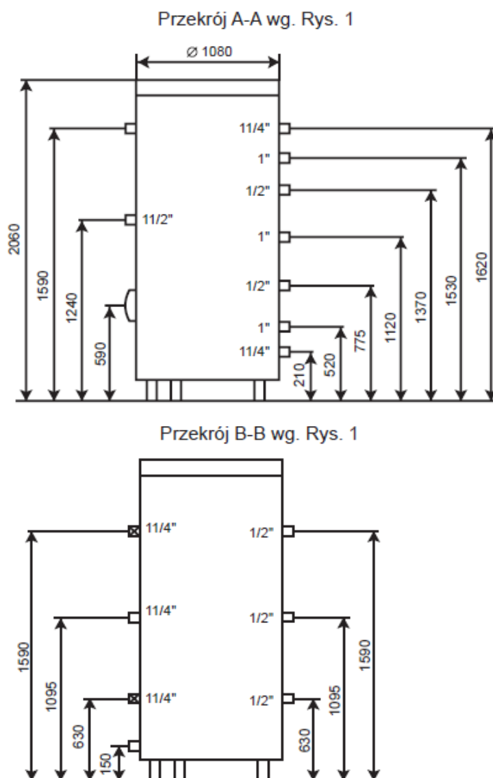
Rys. 2 Wymiary podgrzewacza
