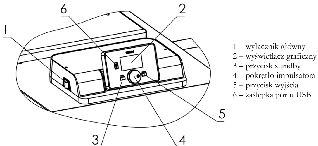
Rys. 2. Panel sterujący sterownika EL 483 zPID
