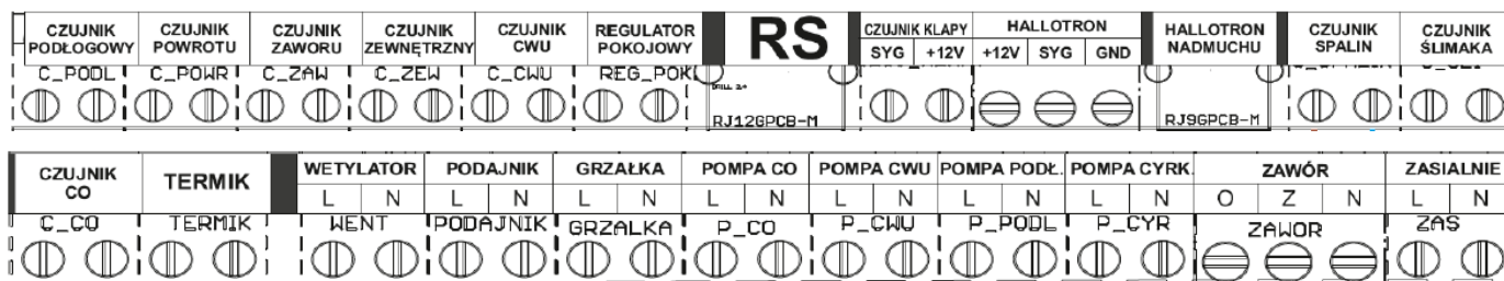
Rys. 3 Listwa przyłączeniowa sterownika El 483 zPID
