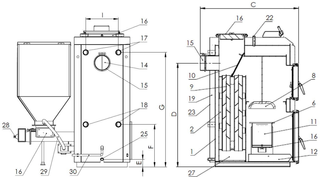
Rys. 1. Konstrukcja i wymiary kotłów EKO-KWP V
