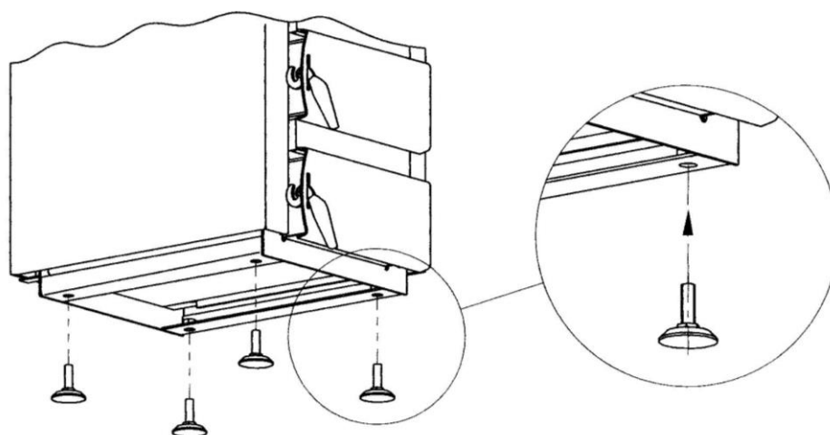
Rys. 6. Poziomowanie kotła
