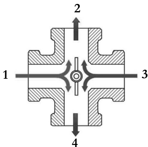
Rys. 8. Czterodrogowy zawór mieszający
