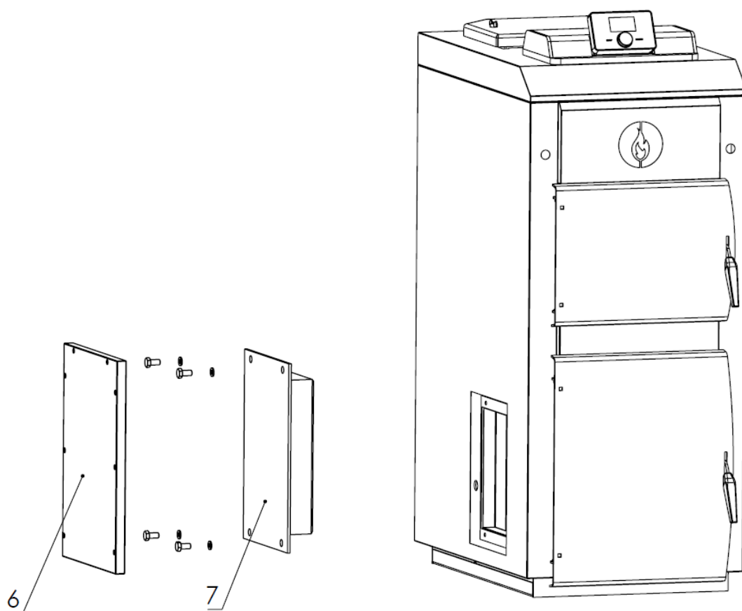
Rys. 4c. Osłona i pokrywa otworu retorty
