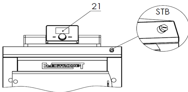
Rys.4b. Termostat bezpieczeństwa STB Sterownik EL 483 zPID
