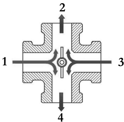
Rys. 7. Czterodrogowy zawór mieszający
