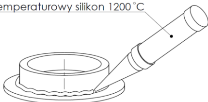
Rys. 12b. Przygotowanie pierścienia
