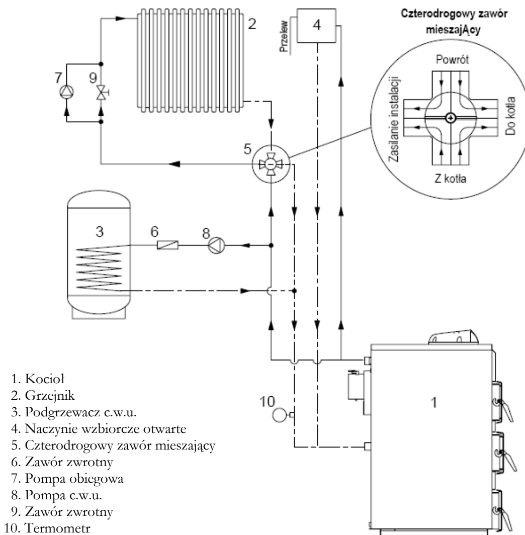
Rys. 9. Przykładowy schemat podłączenia kotła do systemu grzewczego c.o. i c.w.u. z wykorzystaniem czterodrożnego zaworu mieszającego.
