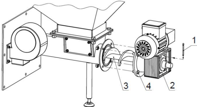
Rys. 13a. Demontaż ślimaka z podajnika kotła. palnika retortowego
