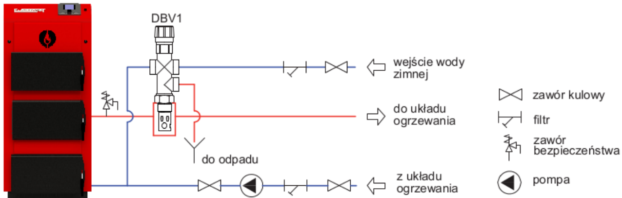
Rys.6 Schemat instalacji z dwudrogowym zaworem bezpieczeństwa DBV1.
