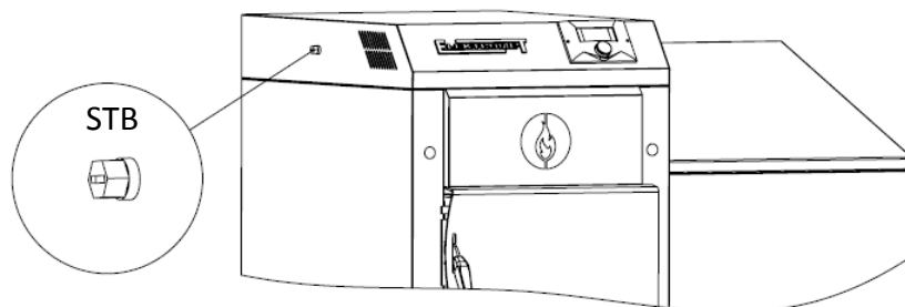
Rys.4a. Termostat bezpieczeństwa STB Sterownik EL 480 zPID
