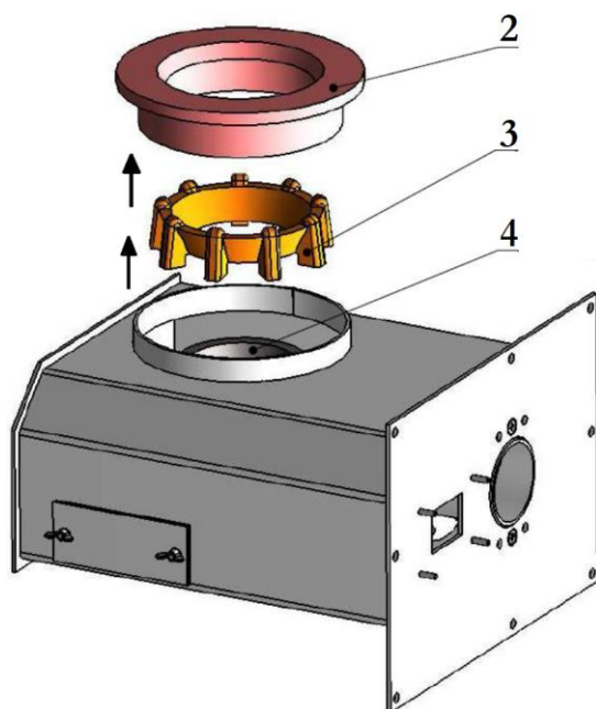
Rys. 12a. Demontaż palnika retortowego
