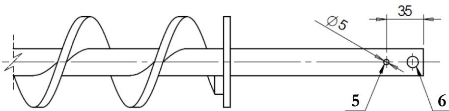
Rys. 13a. Demontaż ślimaka z podajnika kotła. palnika retortowego
