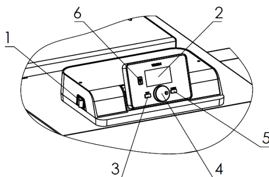
Rys. 2a. Panel sterujący sterownika EL 483 zPID
