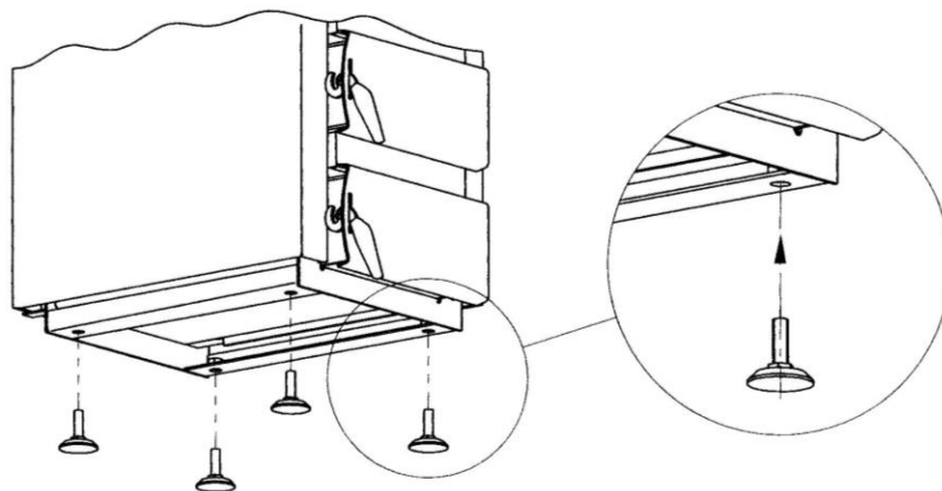
Rys. 5. Pозиomowanie kotła
