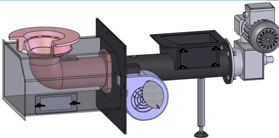
Rys. 15. Pogląd układu podawania i spalania paliwa
