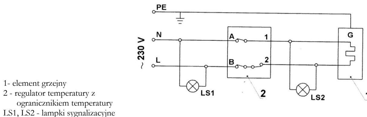
Rys.6 Schemat instalacji elektrycznej ogrzewacza NORDIC 2000
