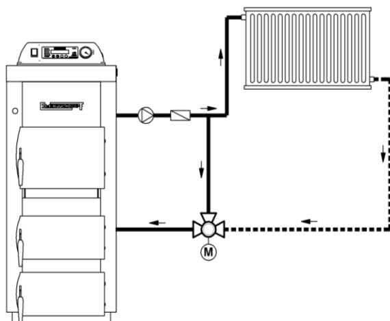
Rys. 7a. Przykład montażu zaworu mieszającego w instalacji z regulacją ilościową (zapewnia ochronę kotła przed „zimnym” powrotem czynnika grzewczego).
