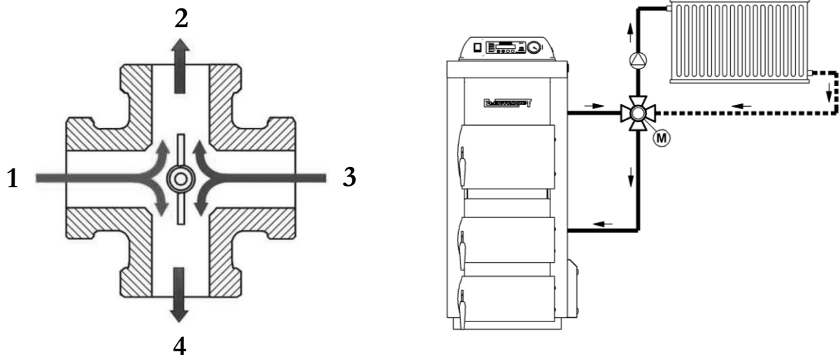
Rys. 6. Czterodrogowy zawór mieszający
