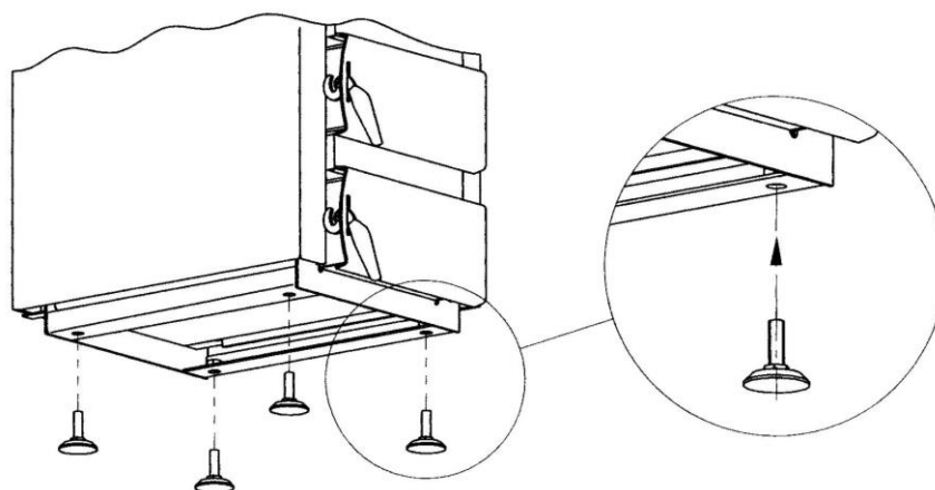
Rys. 4. Pозиomowanie kotła
