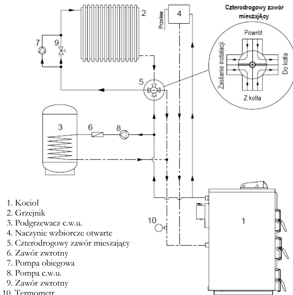
Rys. 8. Przykładowy schemat podłączenia kotła do systemu grzewczego c.o. i c.w.u. z wykorzystaniem czterodrogowego zaworu mieszającego.
