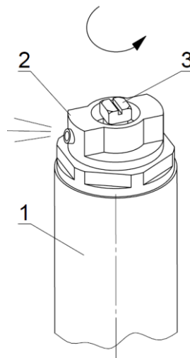
Rys.9. Odpowietrznik 1 – rura odpowietrznika 2 – odpowietrznik 3 – wkręt
