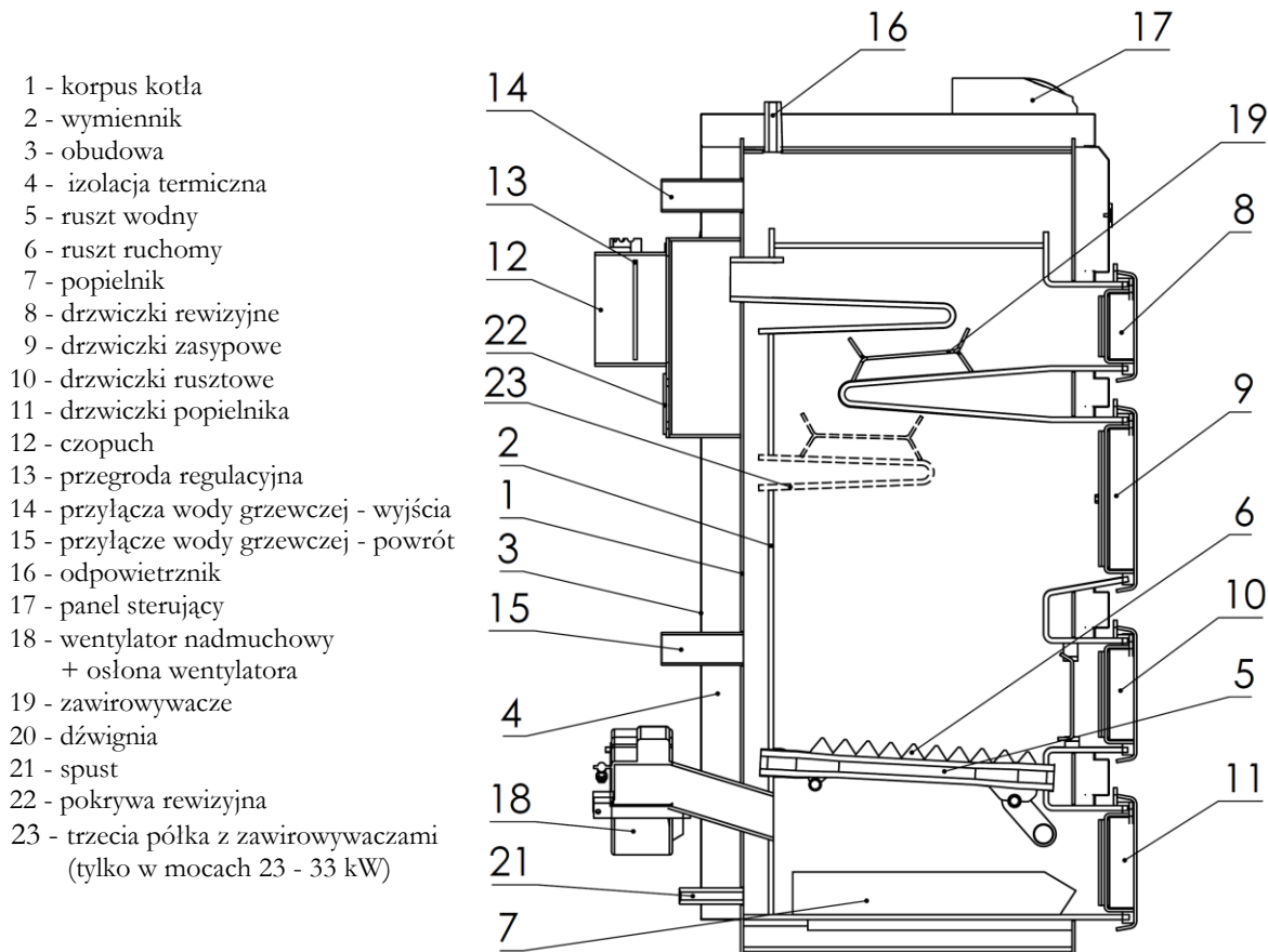
Rys. 1. Schemat konstrukcji kotłów typ EKO-KWW STRONG
