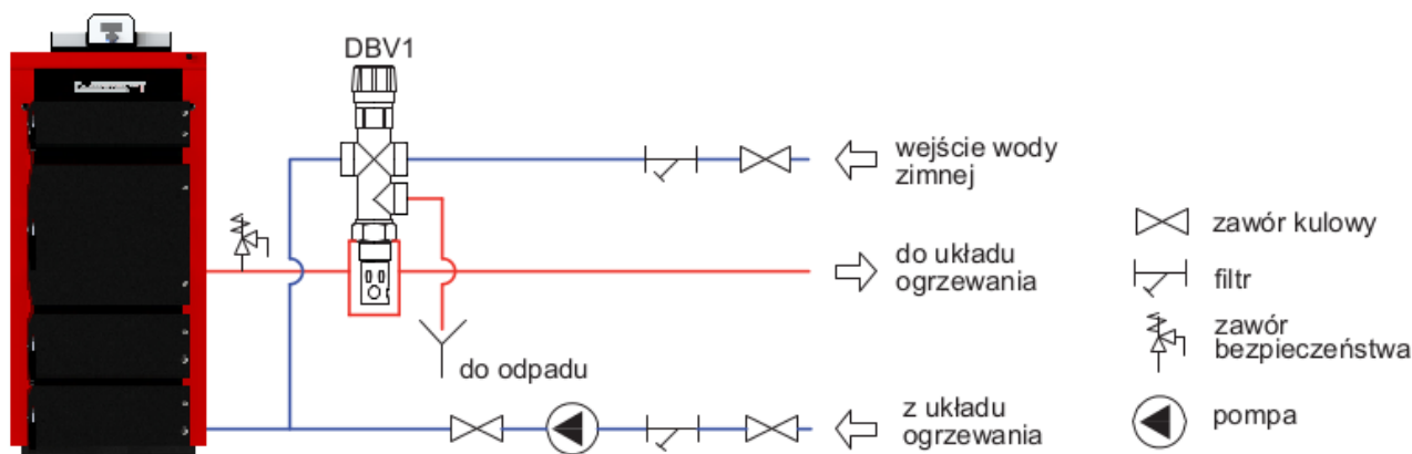
Rys.7 Schemat instalacji z dwudrogowym zaworem bezpieczeństwa DBV1.
