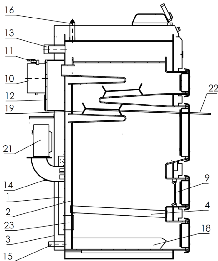
Rys. 1b. Schemat konstrukcji kotłów typ EKO-KWW 23-33
