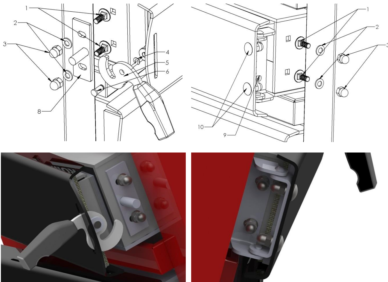
Rys. 5. Przekładanie drzwiczek
