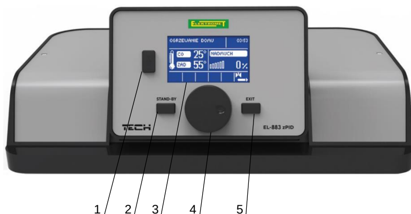
Rys. 4. Panel sterownika EL883 zPID
