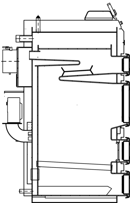
Rys. 1a. Schemat konstrukcji kotłów typ EKO-KWW 14-18
