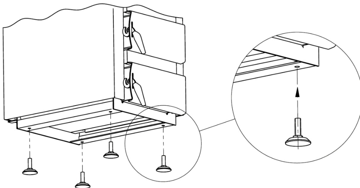
Rys. 6. Pозиomowanie kotła
