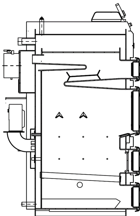
Rys. 1a. Schemat konstrukcji kotłów typ EKO-KWU 14-18
