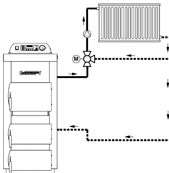
Rys. 9b. Przykład montażu zaworu mieszającego w instalacji z regulacją jakościową (nie zapewnia ochrony kotła przed „zimnym” powrotem czynnika grzewczego).
