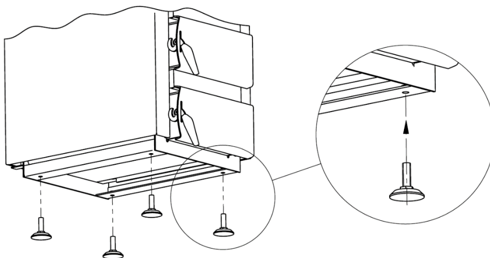
Rys. 6. Pозиomowanie kotła
