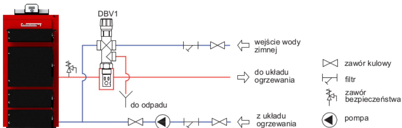
Rys.7 Schemat instalacji z dwudrogowym zaworem bezpieczeństwa DBV1.
