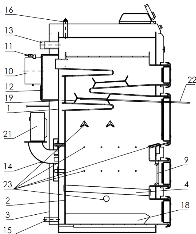
Rys. 1b. Schemat konstrukcji kotłów typ EKO-KWU 23-33
