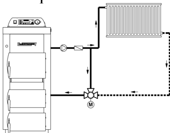
Rys. 11a. Przykład montażu zaworu mieszającego w instalacji z regulacją ilościową (zapewnia ochronę kotła przed „zimnym” powrotem czynnika grzewczego).
