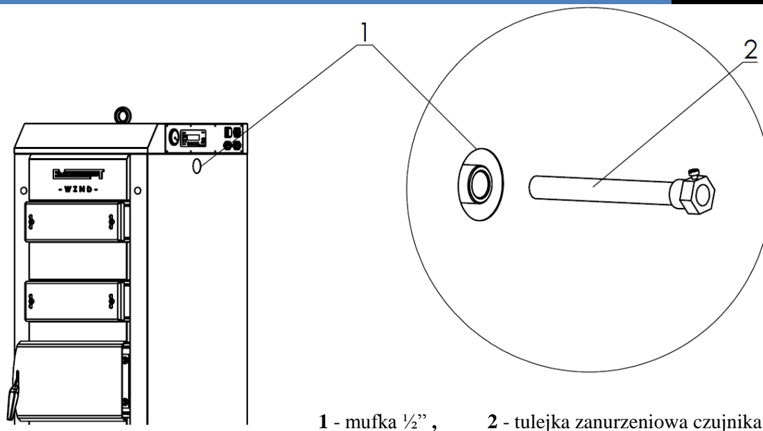
Rys.9 Montaż tulejki zanurzeniowej czujnika zabezpieczenia termicznego.
