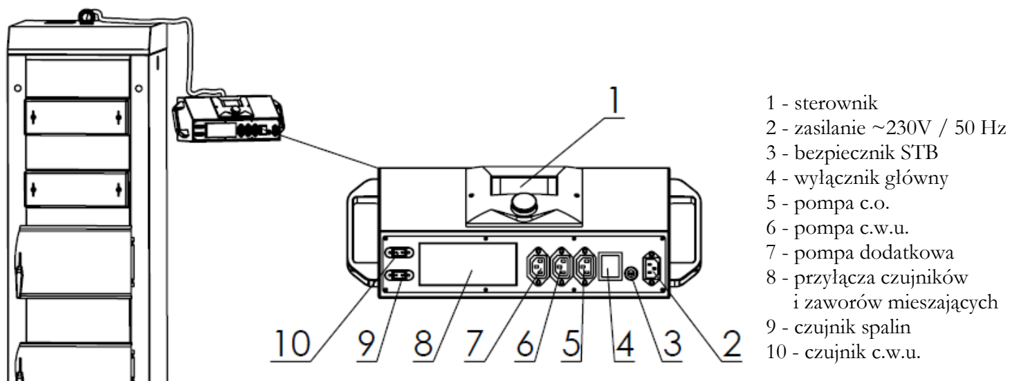
Rys. 3. Przyłącza w listwie sterownika EL 880 zPID.
