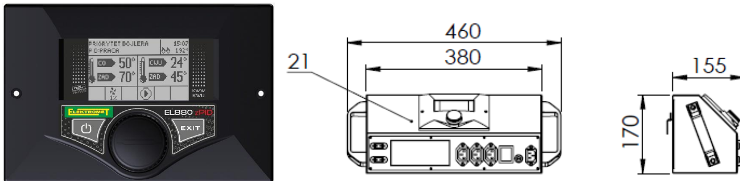
Rys. 4. Wymiary panelu sterownika EL880 zPID.
