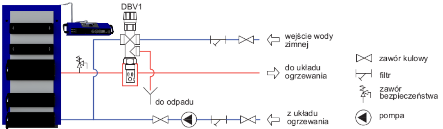
Rys.7 Schemat instalacji z dwudrogowym zaworem bezpieczeństwa DBV1.
