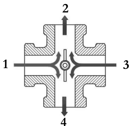
Rys. 10. Czterodrożny zawór mieszający.
