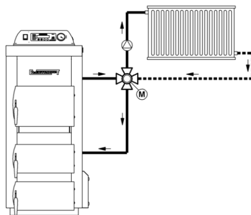
Rys.10a. Przykład montażu zaworu mieszającego czterodrożowego.
