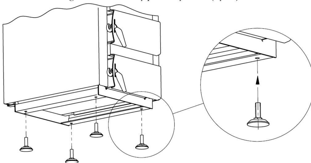
Rys. 6. Poziomowanie kotła.
