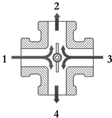
Rys. 5. Czterodrożny zawór mieszający 1 - zasilanie z kotła 3 - powrót z instalacji 2 - zasilanie instalacji 4 - powrót do kotła
