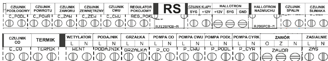
Rys. 2b. Listwa przyłączeniowa sterownika El 483 zPID
