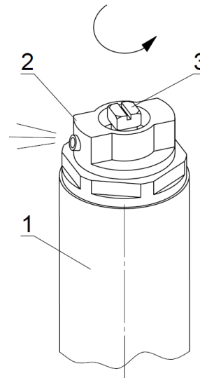
Rys.8. Odpowietrznik 1 - rura odpowietrznika 2 – odpowietrznik 3 - wkręt.
