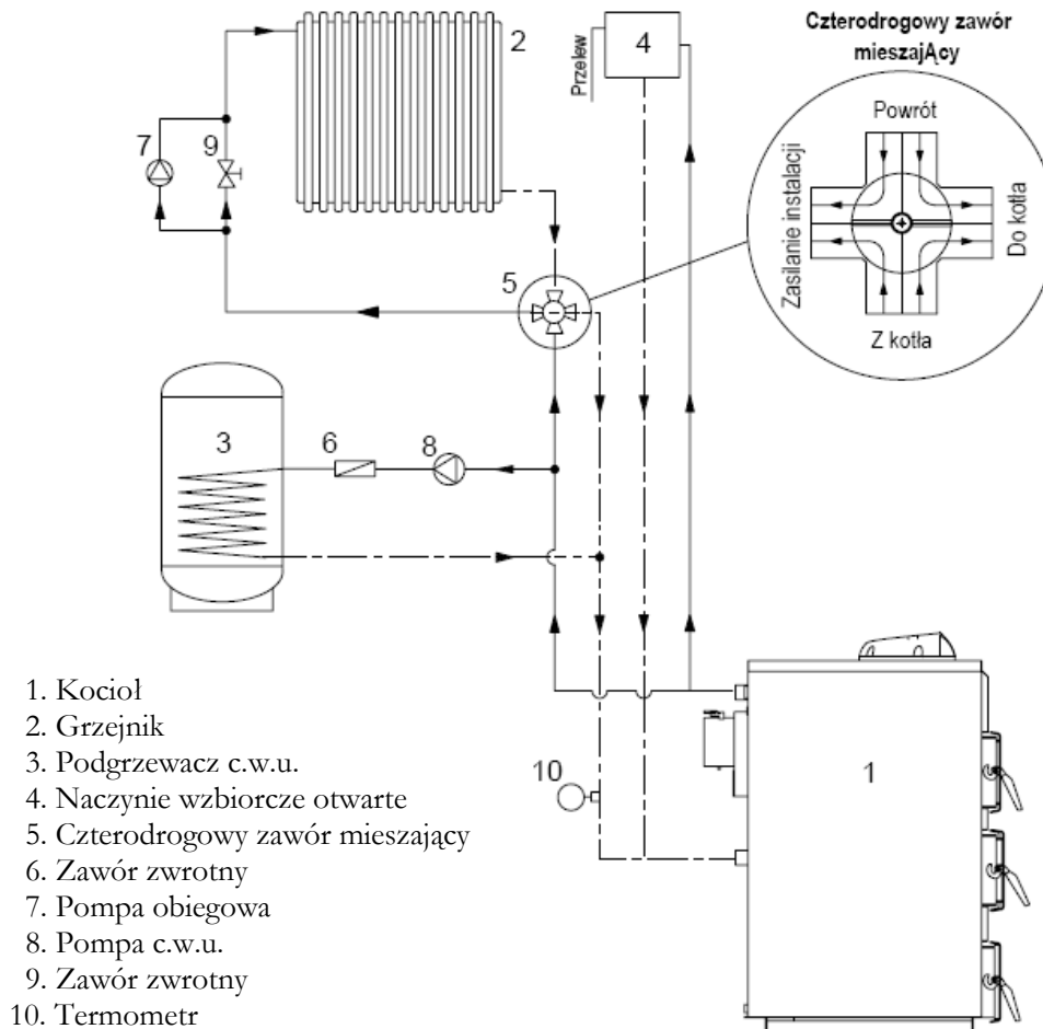
Rys. 7. Przykładowy schemat podłączenia kotła do systemu grzewczego c.o. i c.w.u. z wykorzystaniem czterodrogowego zaworu mieszającego.
