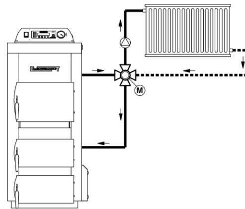
Rys.5a. Przykład montażu zaworu mieszającego czterodrożowego
