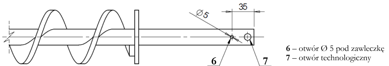
Rys. 14a. Demontaż ślimaka z podajnika kotła. palnika retortowego
