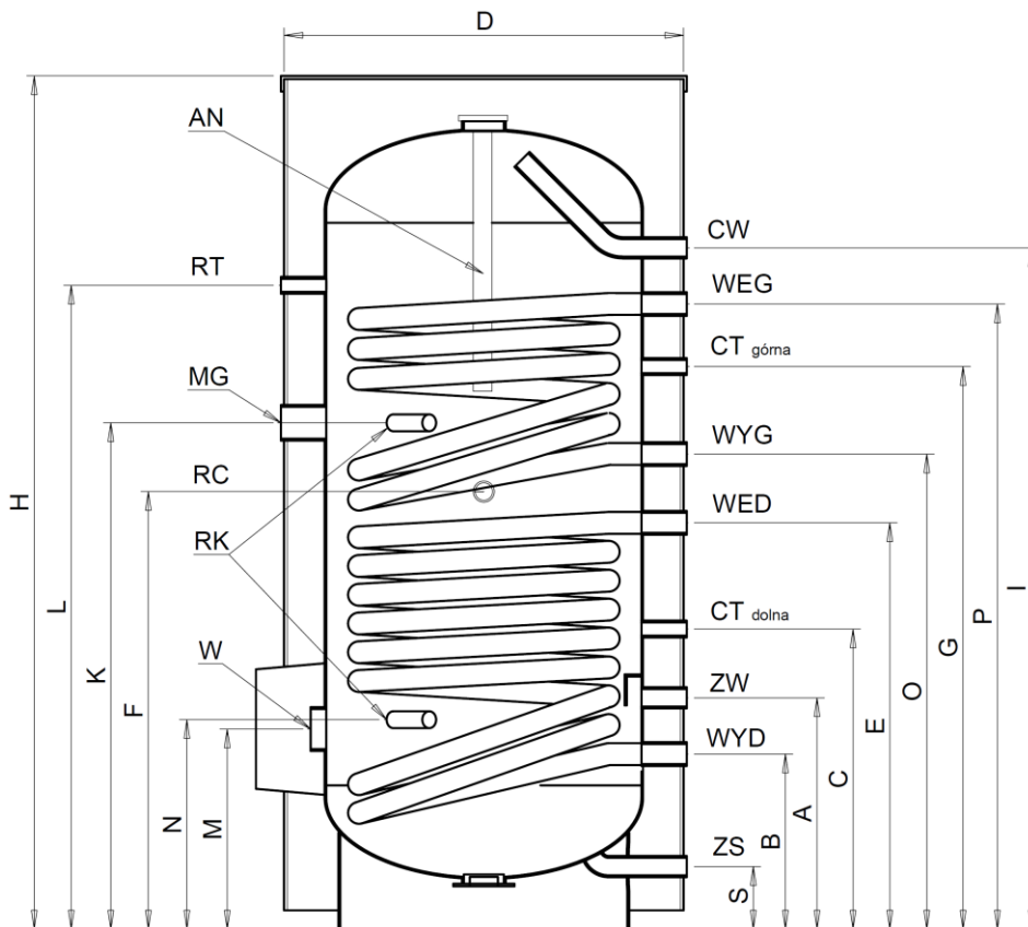
Rys.4 Budowa wymienników WGJ-S 220 DUO FIT
