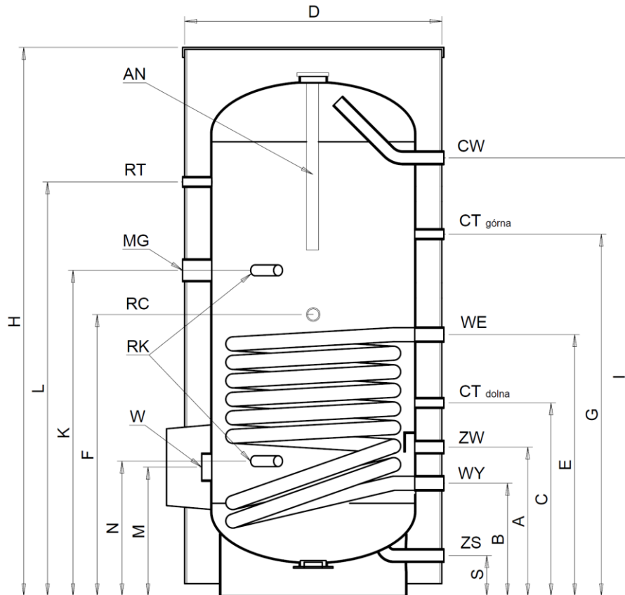
Rys.2 Budowa wymienników WGJ-S 220 FIT
