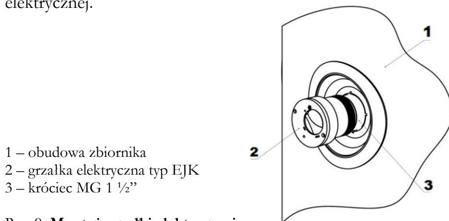
Rys. 9 Montaż grzałki elektrycznej
