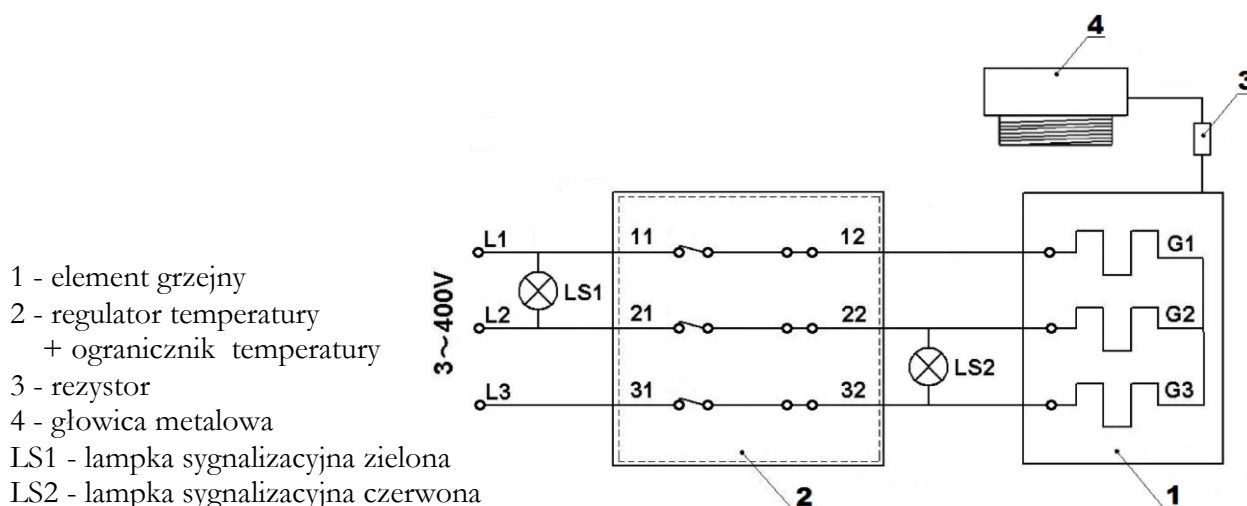
Rys. 11 Schemat elektryczny podgrzewacza z grzałką elektryczną 3- fazową
