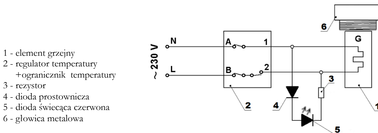
Rys. 10 Schemat elektryczny podgrzewacza z grzałką elektryczną 1- fazową
