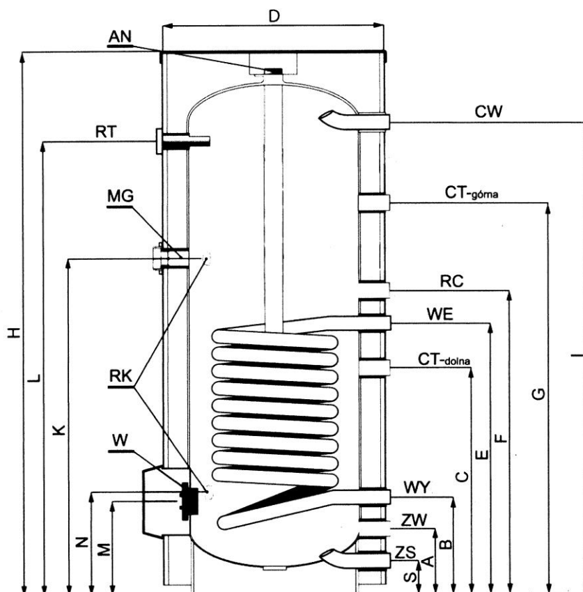
Rys.3 Budowa wymienników WGJ-S 250- 500
