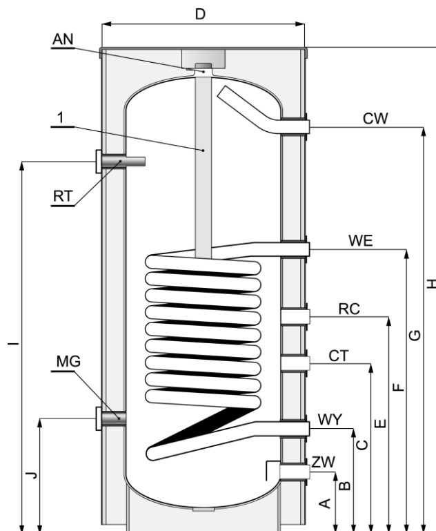
Rys. 1. Budowa wymienników WGJ-S 100 - 150
