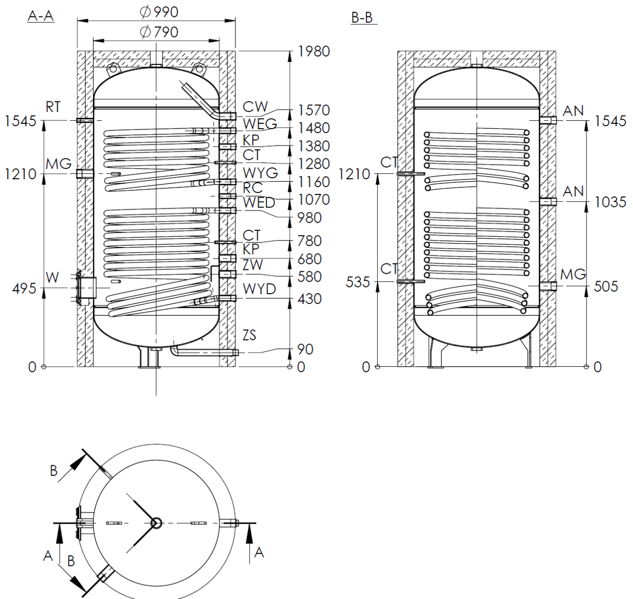
Rys.1 Budowa podgrzewacza WGJ- S 750 DUO PP
