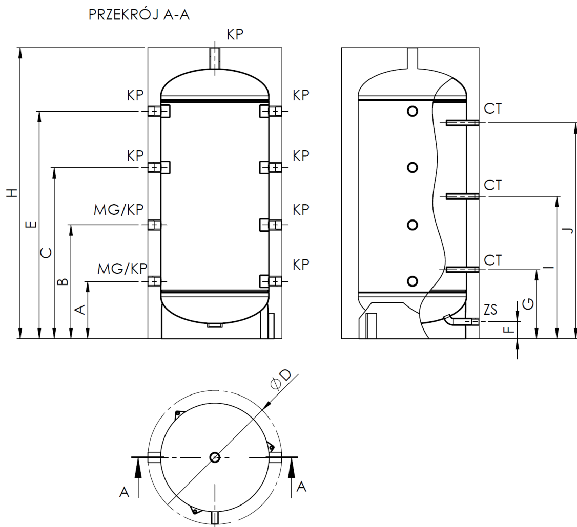
Rys 1. Budowa zbiornika buforowego
