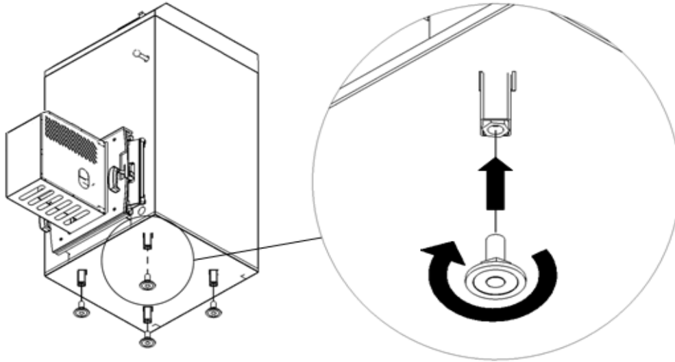
Rys. 4. Poziomowanie kotła
