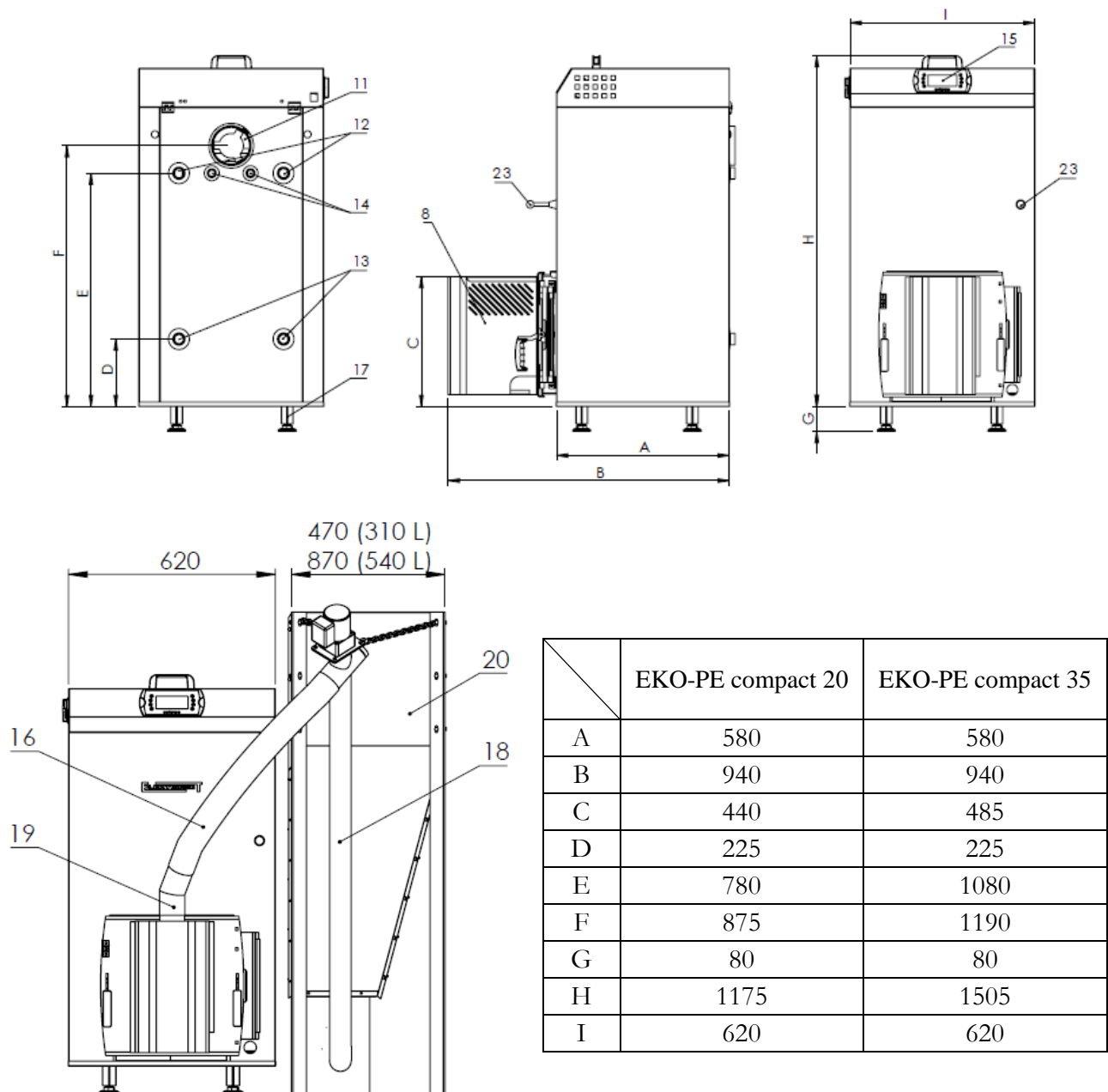
Rys. 1. Budowa i wymiary kotła
