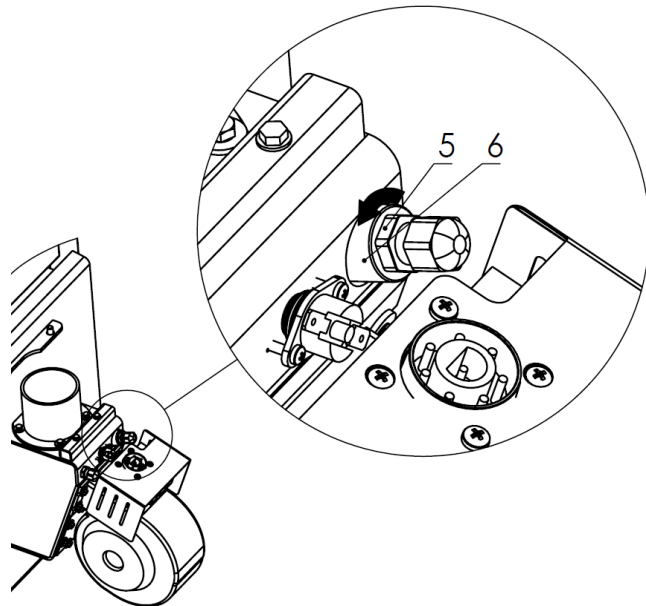
Rys. 18d. Wykręcenie dławicy
