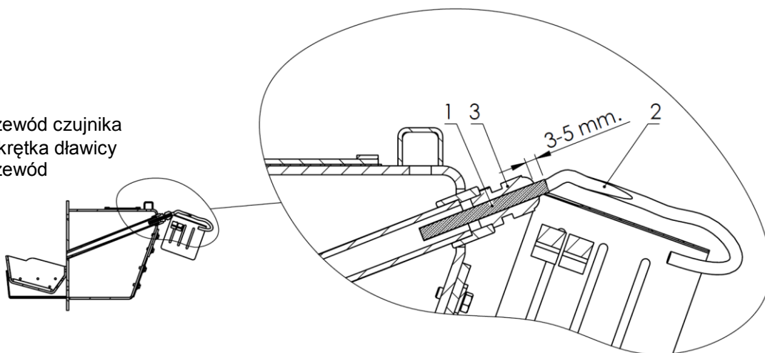
Rys. 19. Osadzenie czujnika
