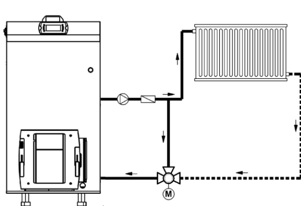
Rys. 9a. Przykład montażu zaworu mieszającego w instalacji z regulacją ilościową (zapewnia ochronę kotła przed „zimnym” powrotem czynnika grzewczego).
