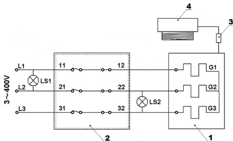
Rys. 4 Schemat elektryczny podgrzewacza z grzałką elektryczną 3- fazową
