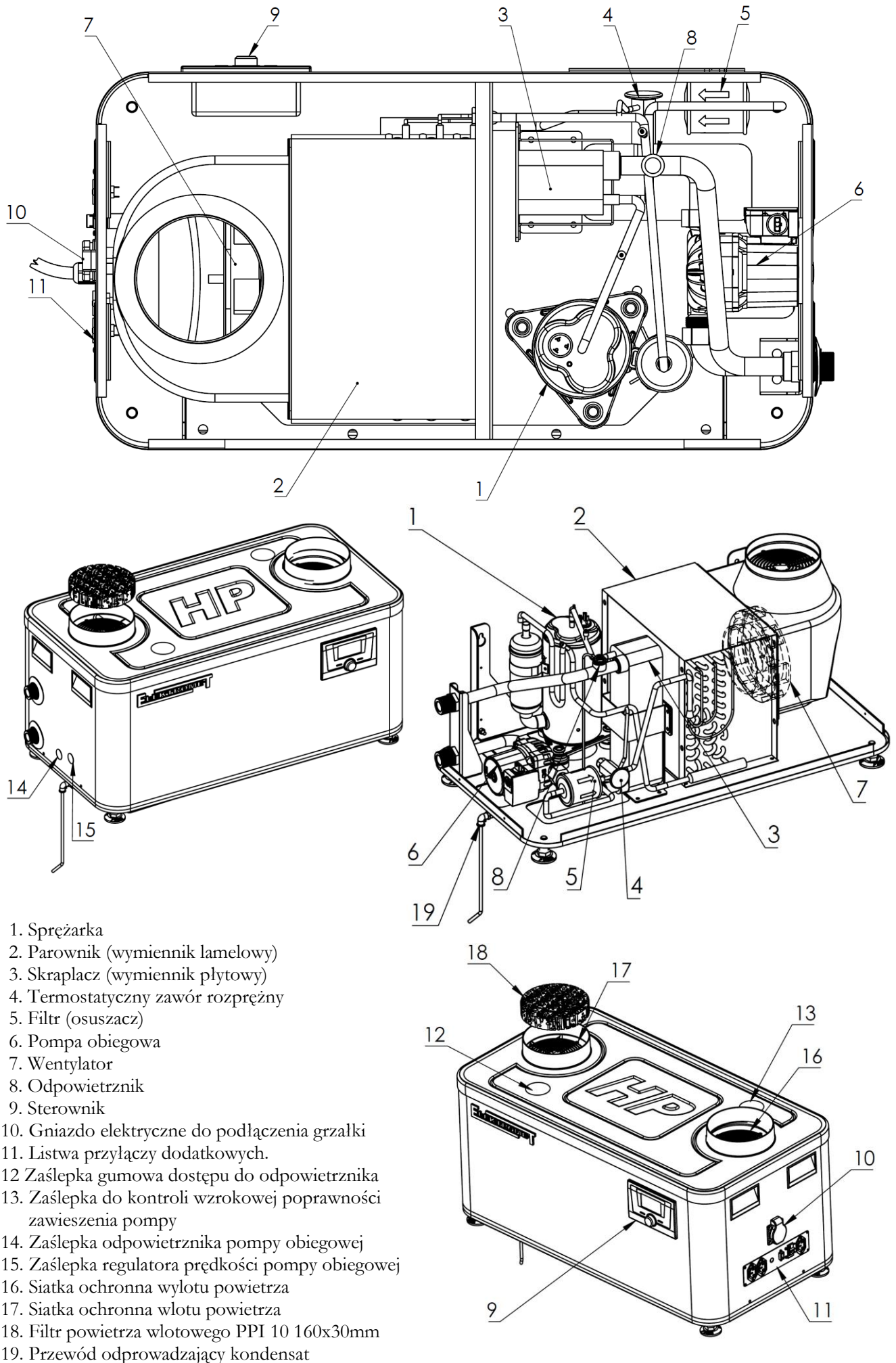
Rys. 2. Budowa pompy ciepła HP ALFA 2.4
