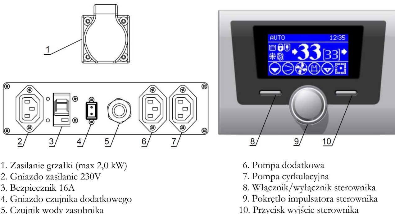
Rys. 3. Listwa przyłączeniowa i panel sterujący sterownika EL-41.
