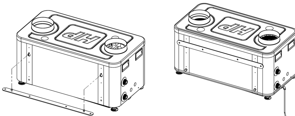
Rys. 5a. Instalacja pompy ciepła na wieszakach.
