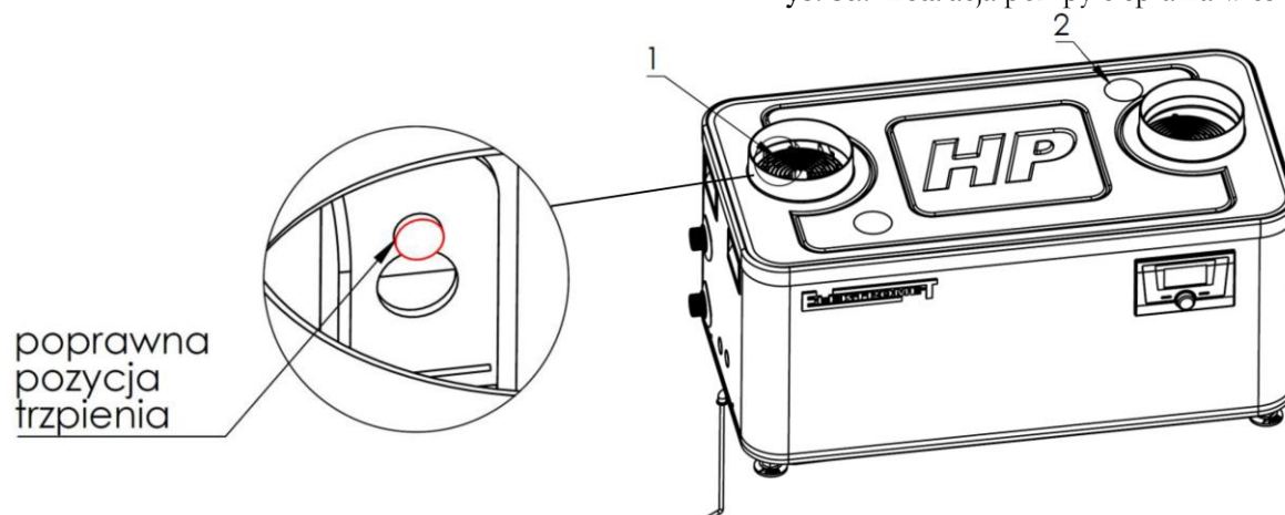
Rys. 5a. Instalacja pompy ciepła na wieszakach.
