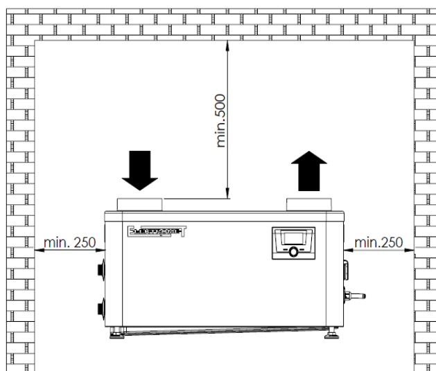
Rys. 4. Instalacja pompy ciepła z zachowaniem niezbędnych odstęgów.
