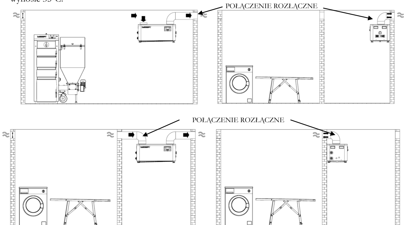
Rys. 8. Przykłady instalacji pompy ciepła.
