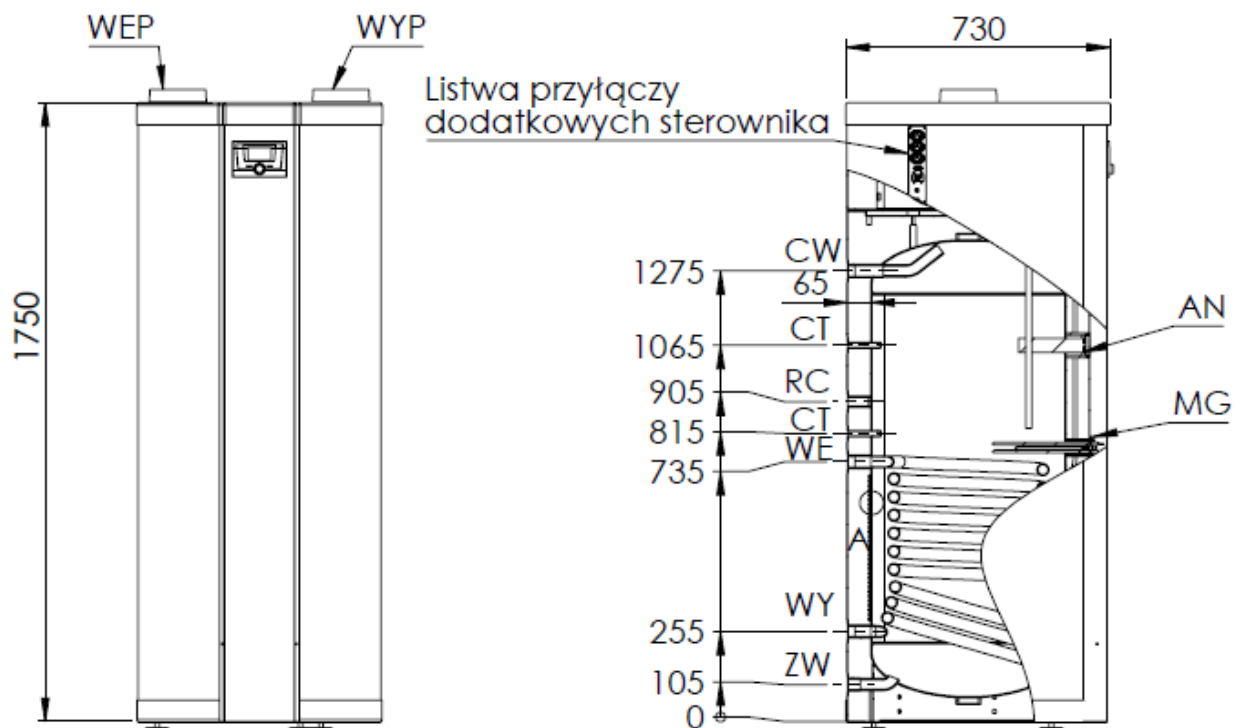
Rys. 1b. Wymiary pompy ciepła WGJ-HP smart 300
