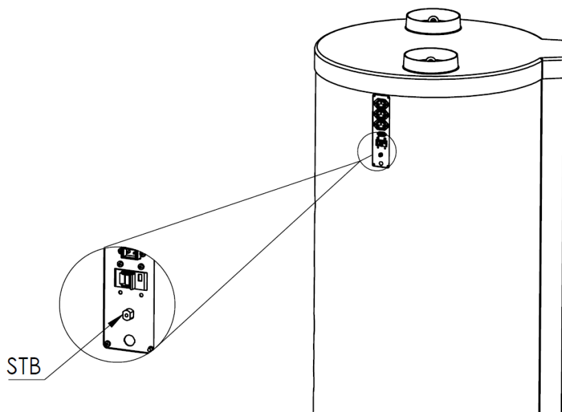
Rys. 3. Niesamoczynny ogranicznik temperatury
