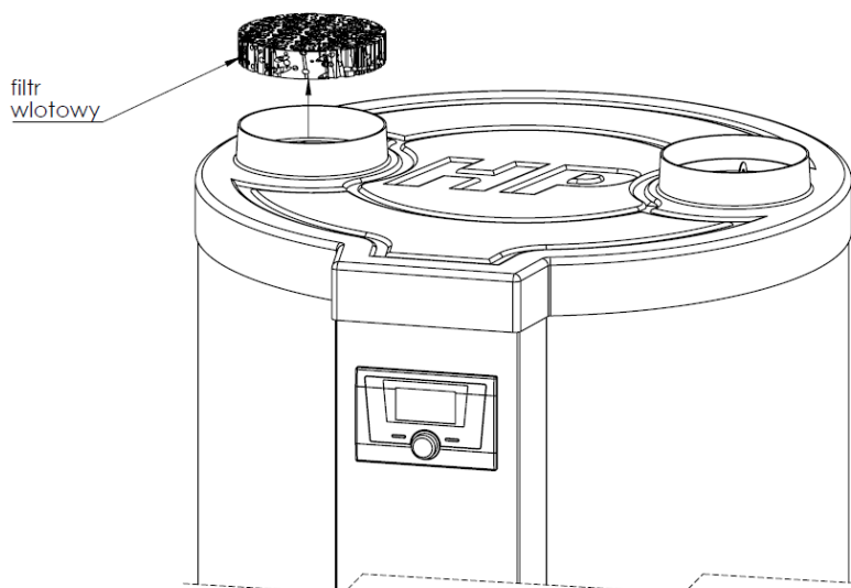
Rys. 8 Umieszczenie filtra wlotowego powietrza
