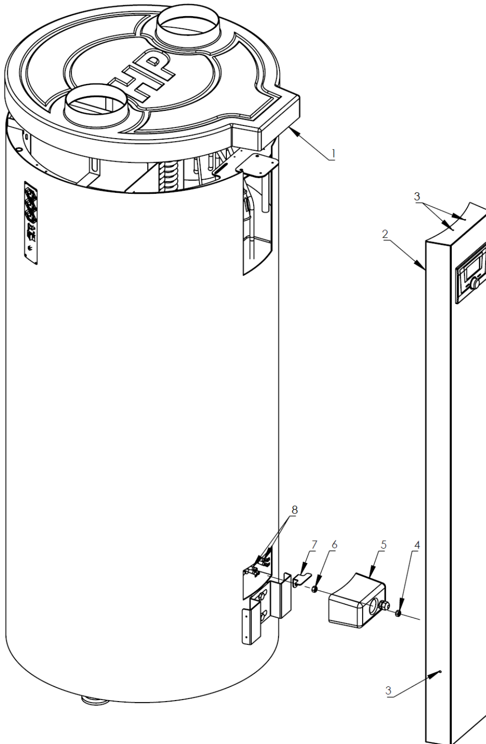
Rys. 9. Demontaż zestawu suchych grzałek elektrycznych.
