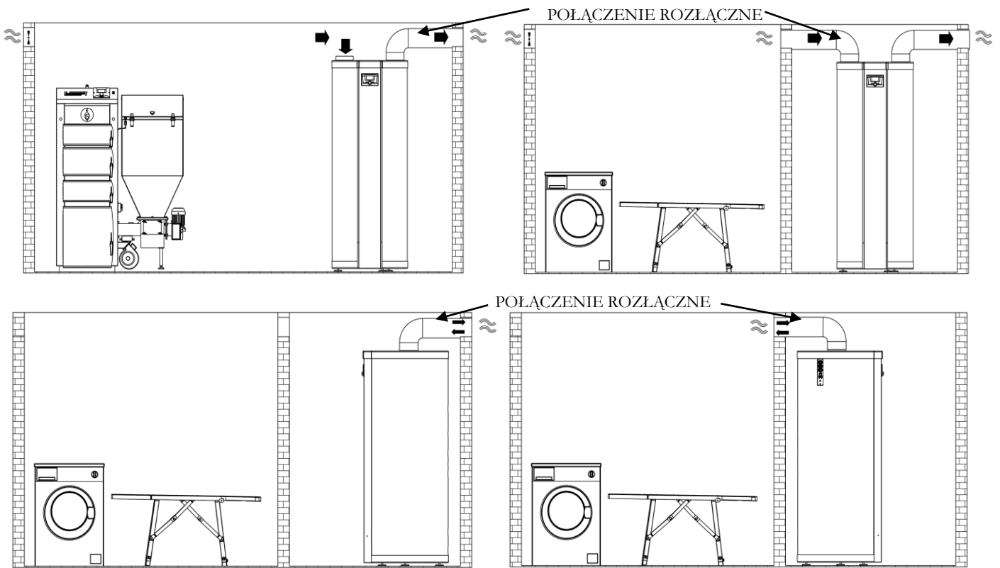
Rys. 6. Przykłady instalacji pompy ciepła
