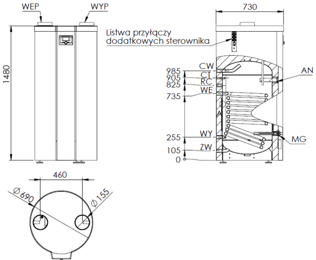
Rys. 1a. Wymiary pompy ciepła WGJ-HP smart 200
