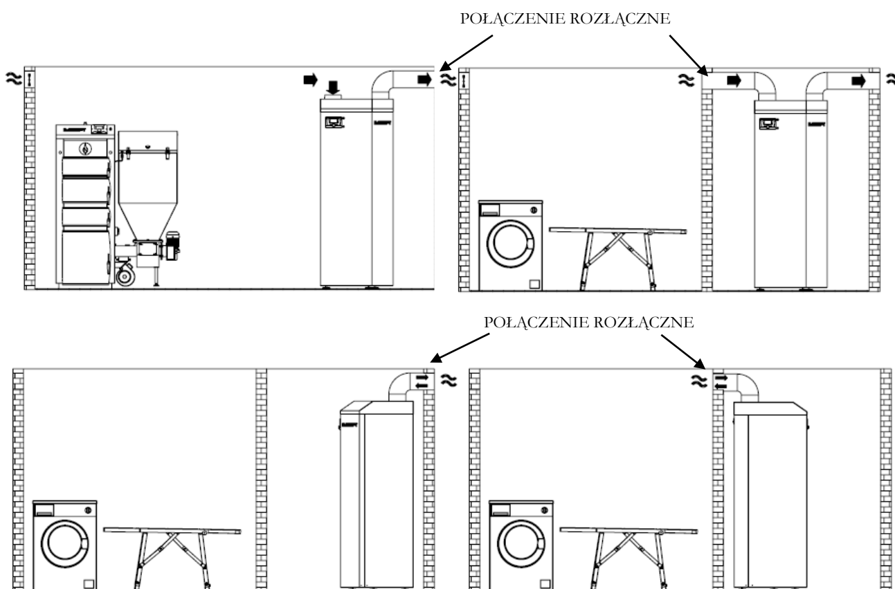
Rys. 6. Przykłady instalacji pompy ciepła
