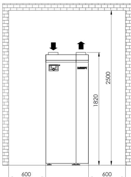
A) Widok z przodu
