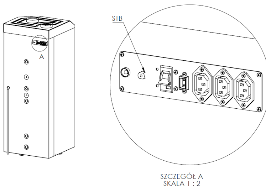
Rys. 3. Niesamoczynny ogranicznik temperatury
