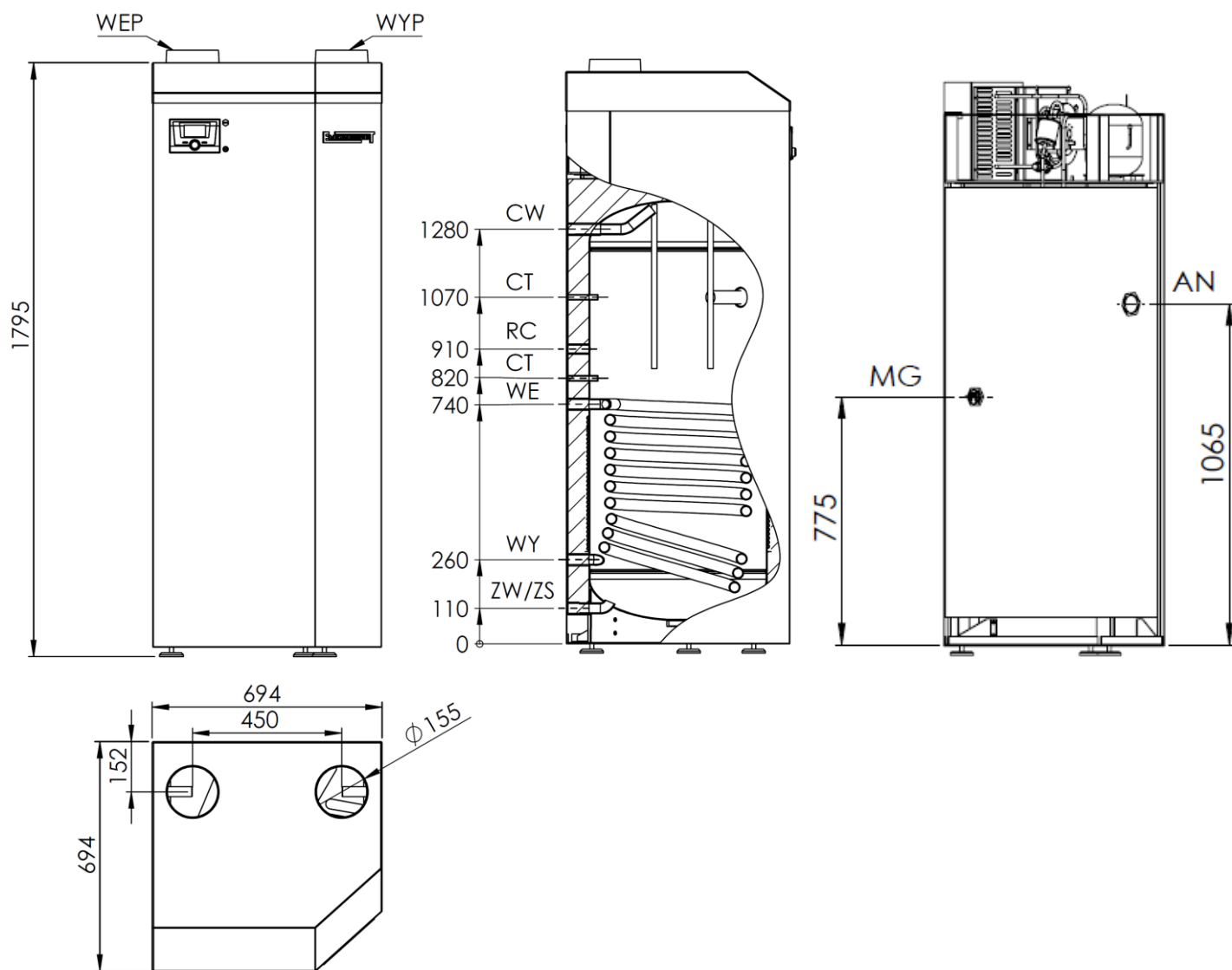
Rys. 1. Wymiary pompy ciepła WGJ-HP
