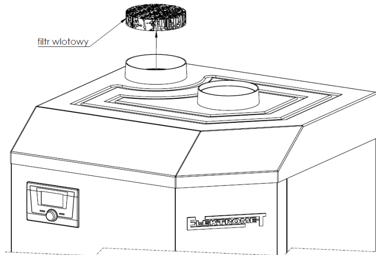
Rys. 8. Umieszczenie filtra wlotowego powietrza
