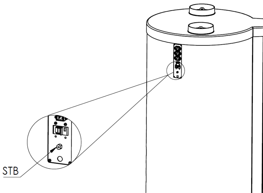
Rys. 3. Niesamoczynny ogranicznik temperatury
