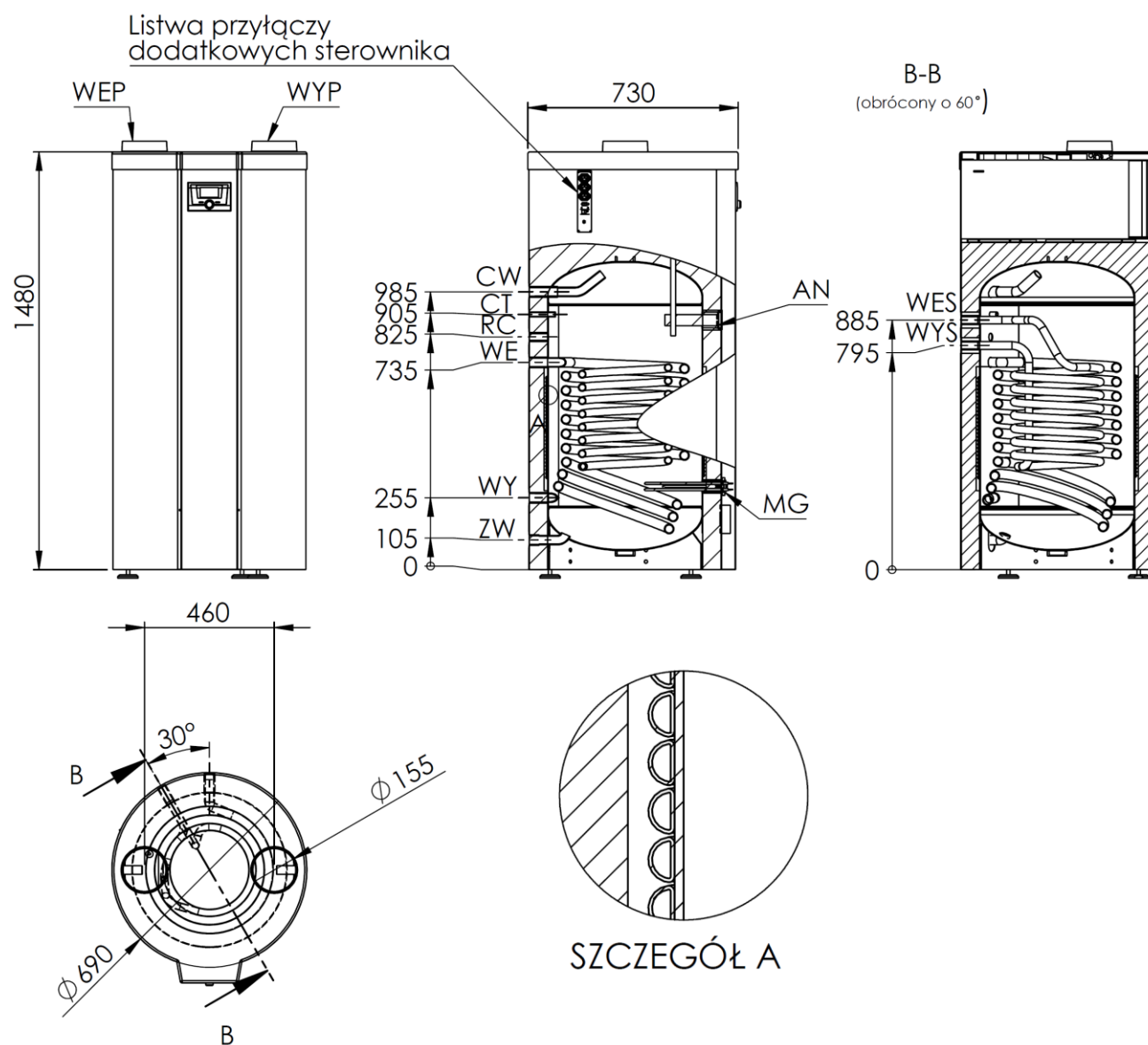
Rys. 1b. Wymiary pompy ciepła WGJ-HP smart 200 DUO
