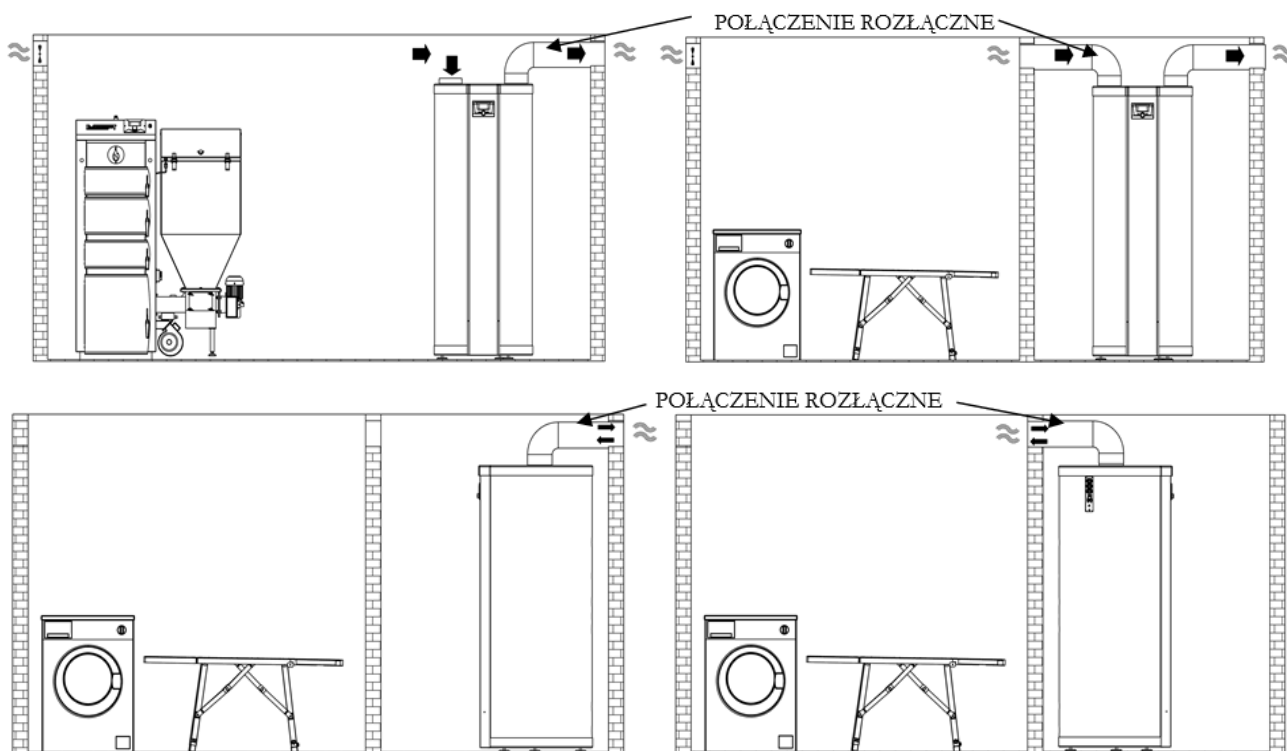
Rys. 6. Przykłady instalacji pompy ciepła
