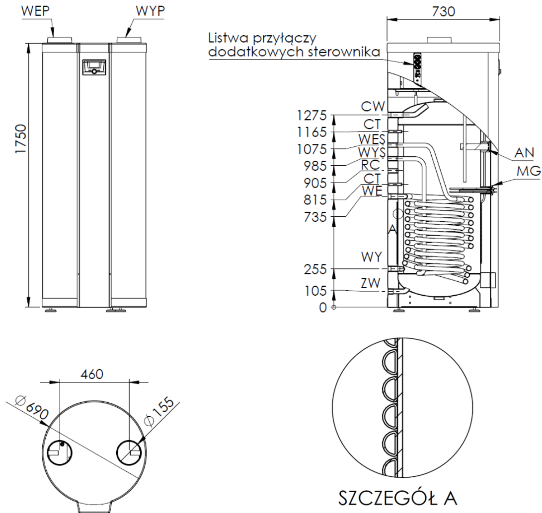
Rys. 1b. Wymiary pompy ciepła WGJ-HP smart 300 DUO
