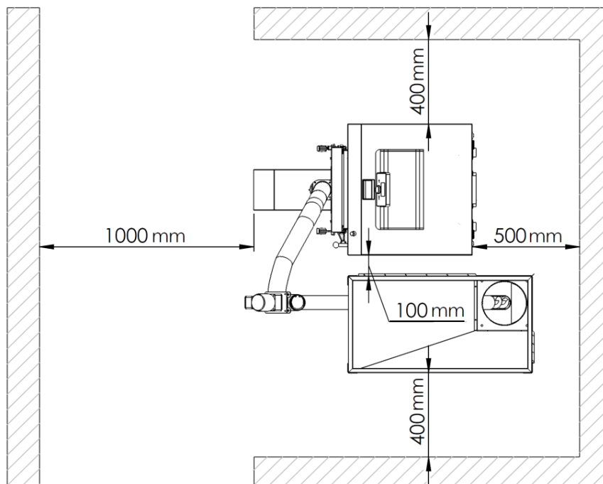
Rys. 5. Ustawienie kotła w kotłowni
