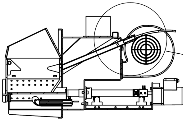
Rys. 22 Osadzenie czujnika
