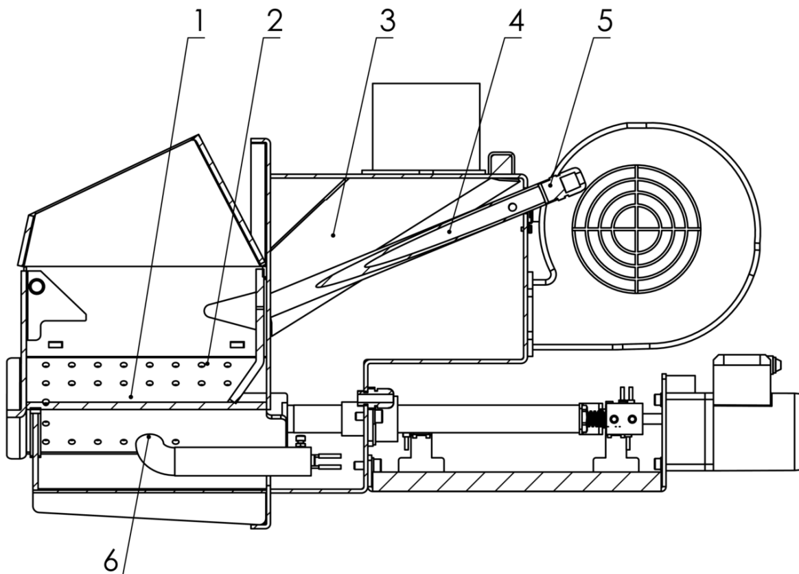
Rys. 20. Czyszczenie palnika
