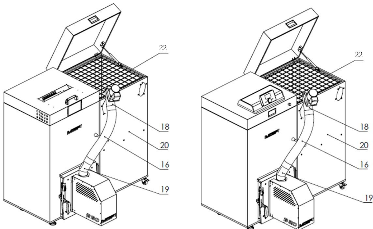
Rys. 1c. Budowa kotła typu EKO-PE mini BOX 20 kW z panelem sterującym IGNEO TOUCH oraz EL-583
