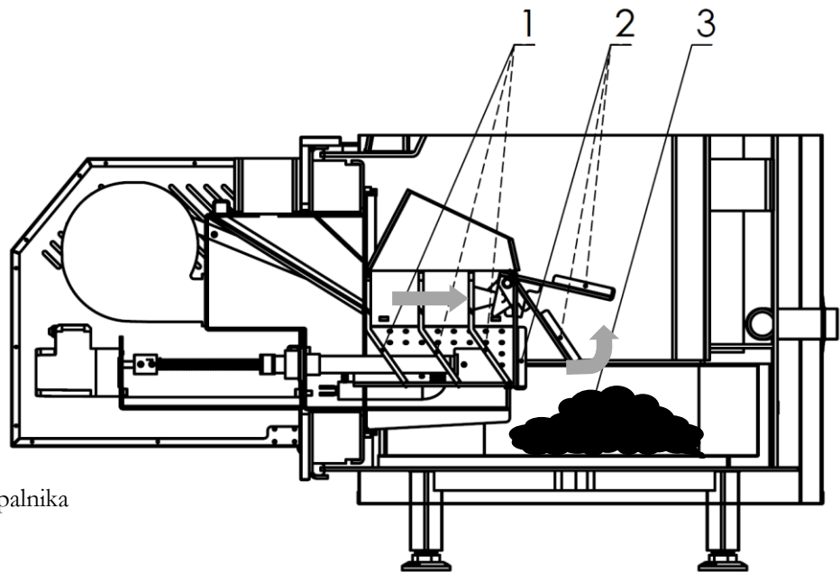
Rys. 24 Układu samoczyszczący palnika
