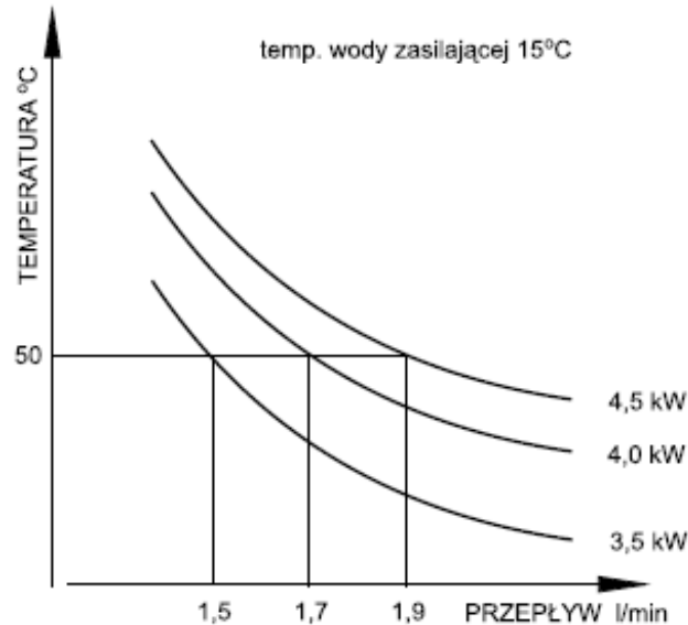
Rys. 2. Zależność temperatury od natężenia przepływu wody
