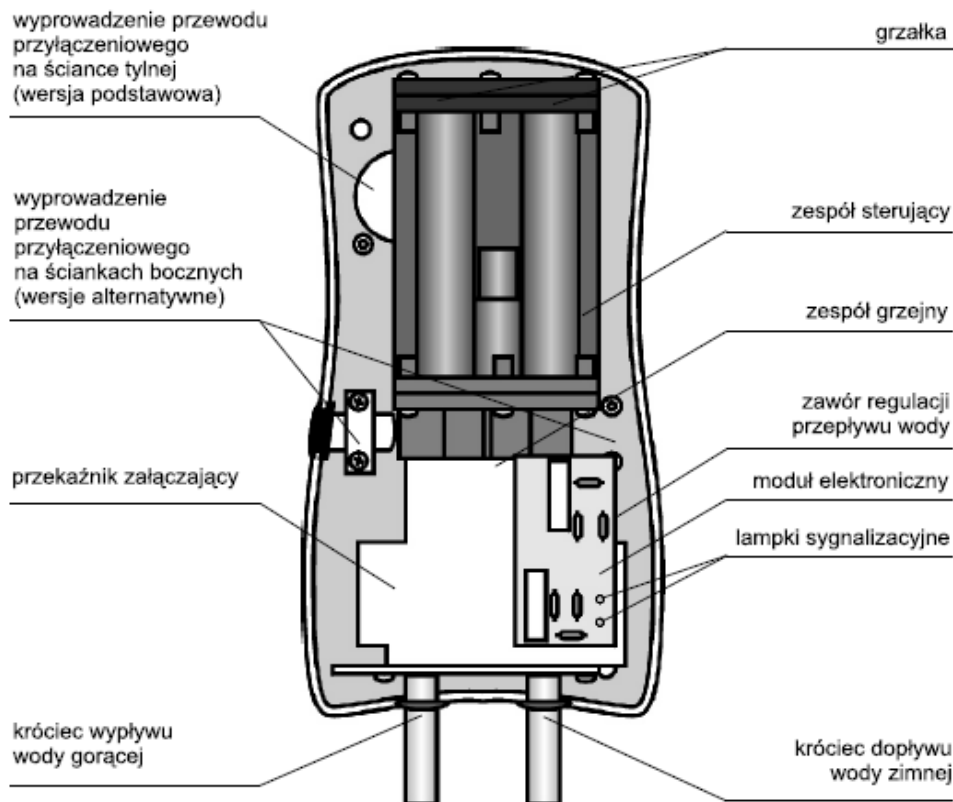
Rys. 1. Budowa Elektrycznego Przepływowego Ogrzewacza Wody - LIDER
