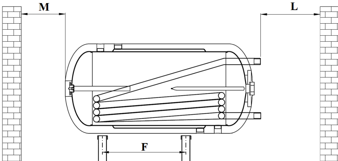
Rys. 3 Instalacja wymiennika dwupłaszczowego.
