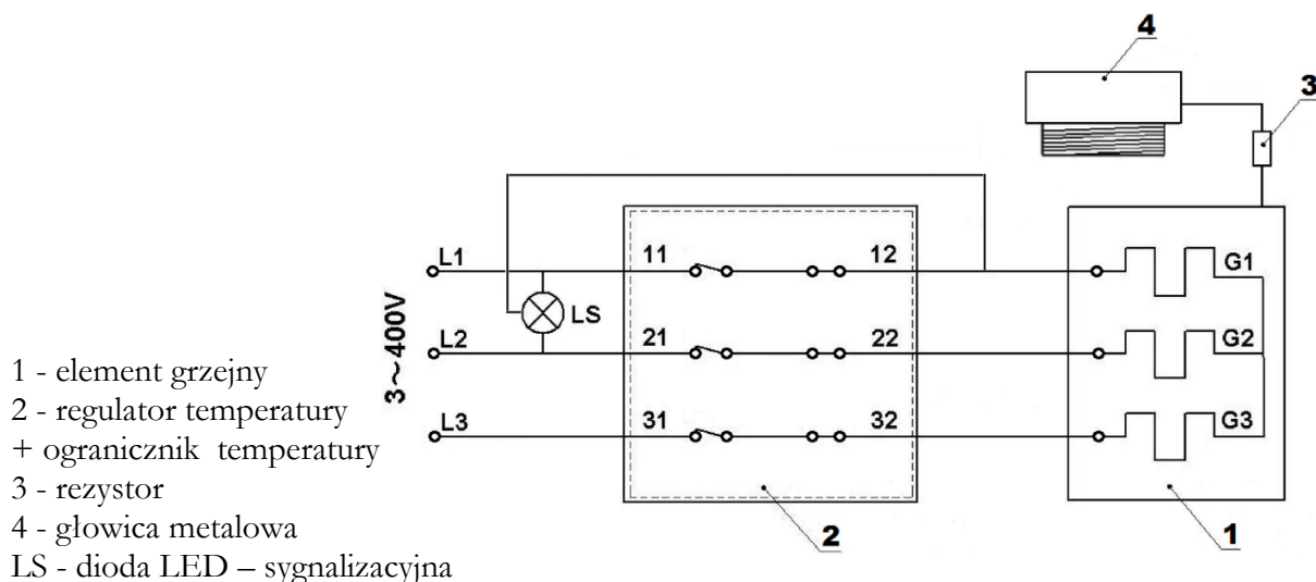
Rys. 3 Schemat instalacji elektrycznej.
