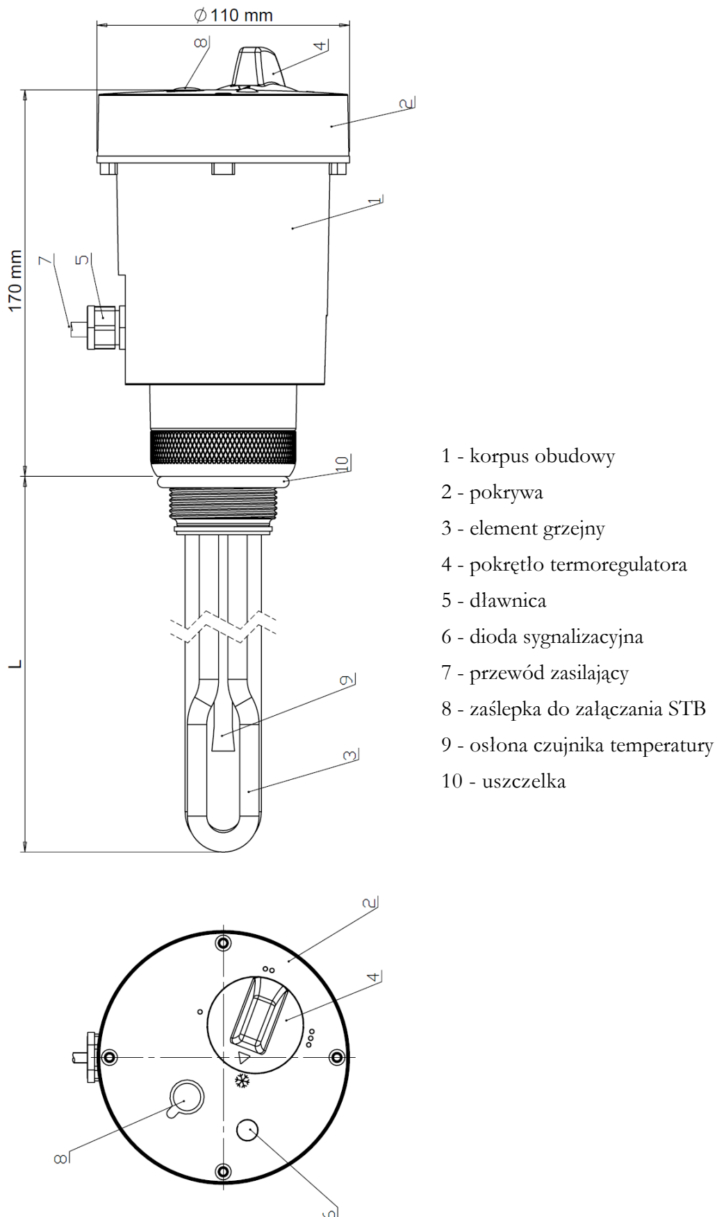
Rys.1 Budowa grzałki.
