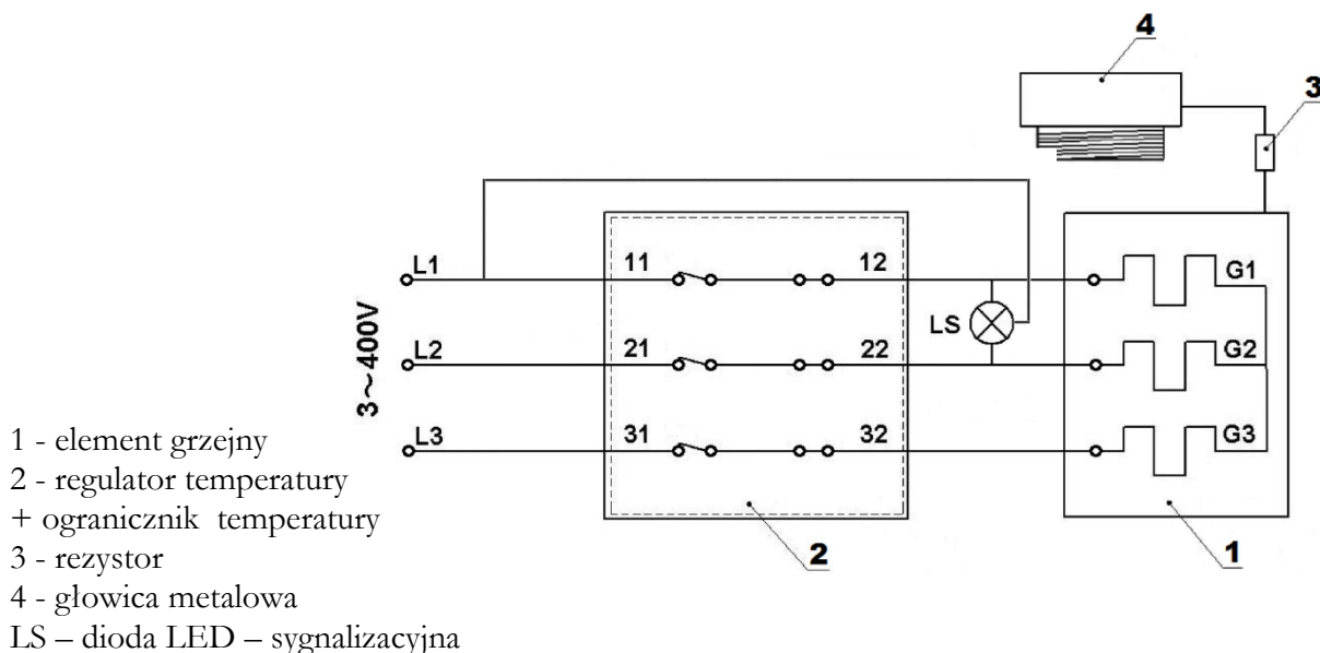
Rys.4 Schemat instalacji elektrycznej grzałki EJK maxi HP ST.
