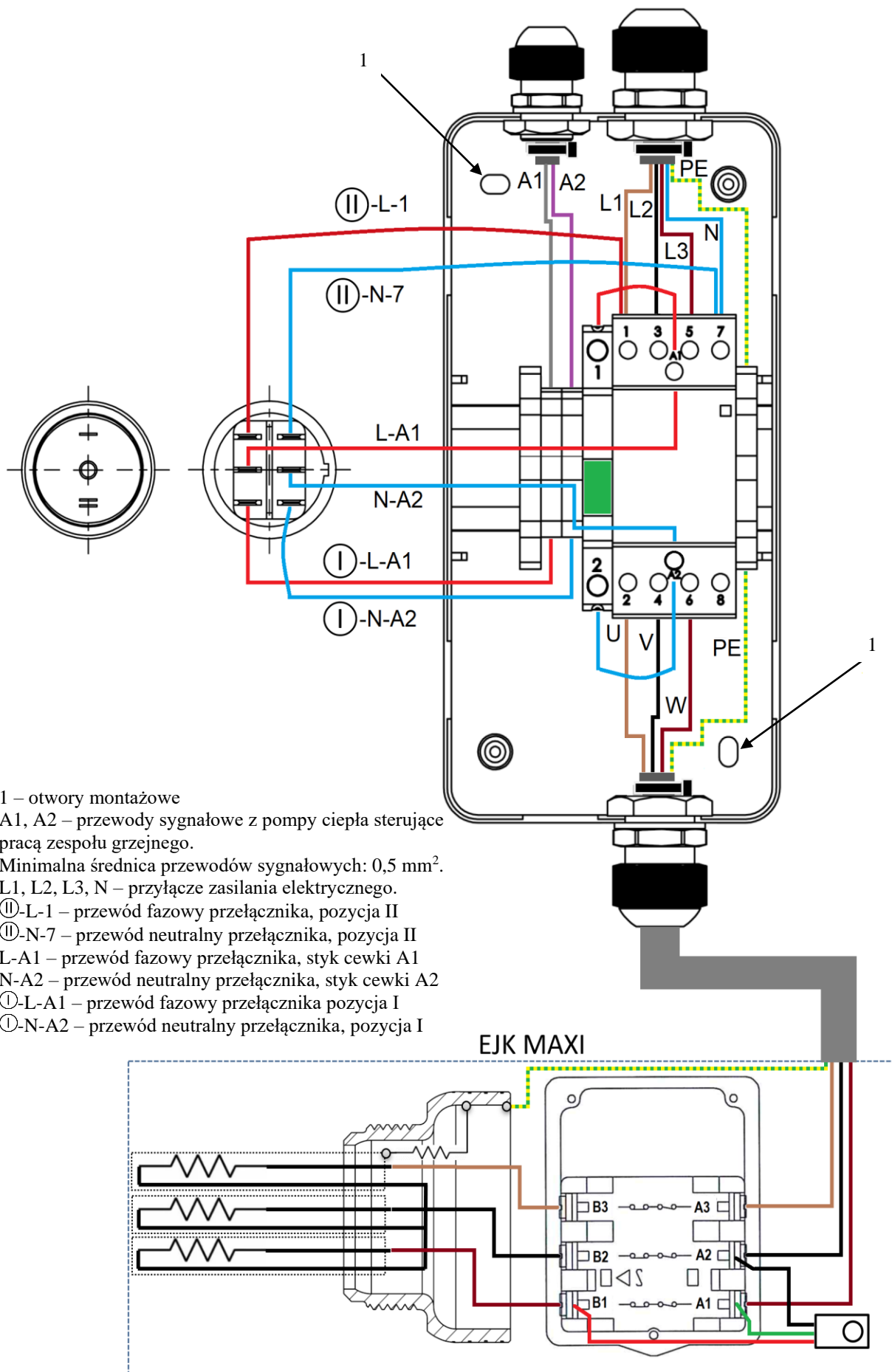
Rys. 5. Podłączenie elektryczne grzałki EJK maxi HP ST.
