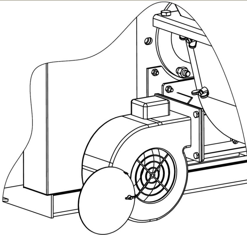
Rys. 21a. Położenie przysłony wentylatora w trybie pracy automatycznej (tj. z wykorzystaniem algorytmu PID).
