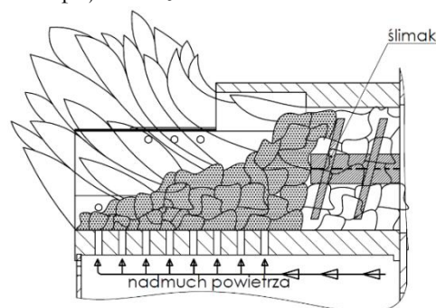
Rys.20 Prawidłowe spalanie
