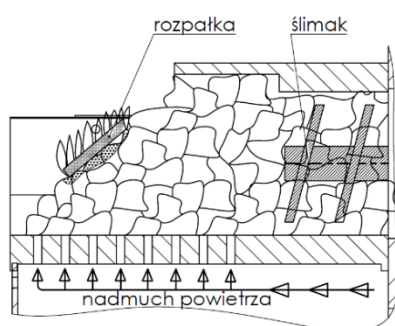
Rys.19 Rozpalanie
