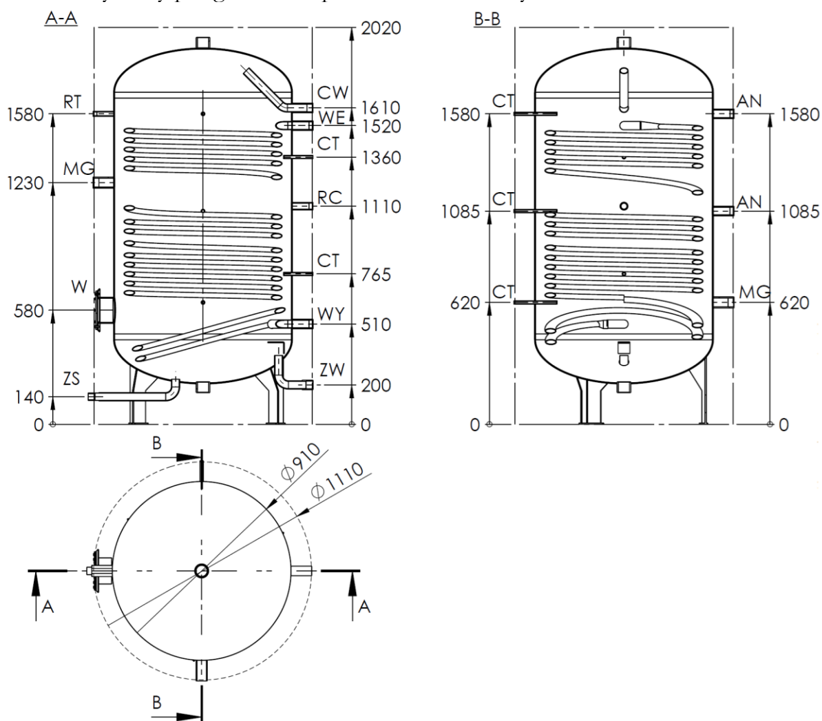
Rys.1 Budowa podgrzewacza WGJ- S 1000/4,8
