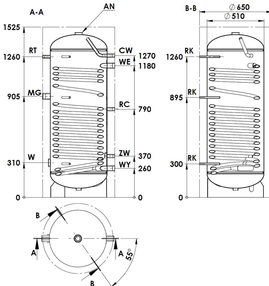
Rys. 2. Budowa wymienników WGJ-S 250 FIT MAX+
