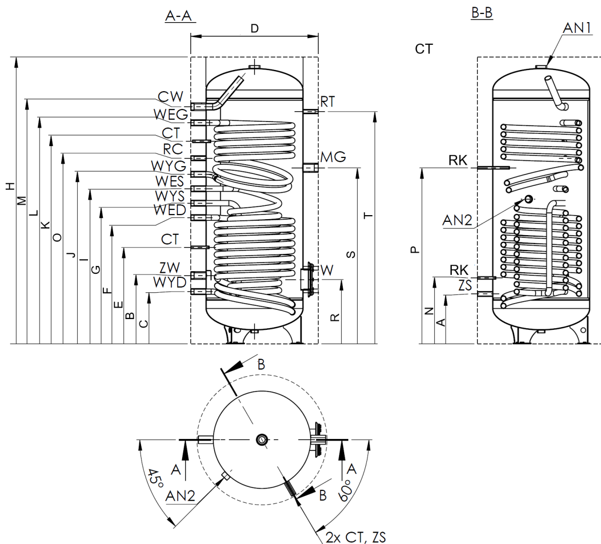
Rys.1 Budowa wymiennika WGJ-S 400 TRIO, WGJ-S 500 TRIO
