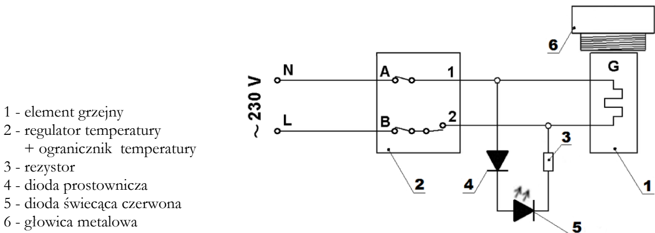
Rys. 5 Schemat elektryczny podgrzewacza z grzałką elektryczną 1- fazową
