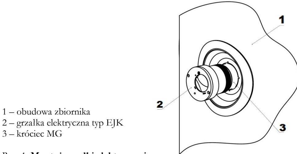
Rys. 4 Montaż grzałki elektrycznej
