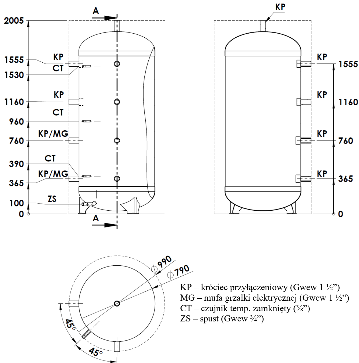
Rys 2. Budowa zbiornika buforowego WGJ-BN 800
