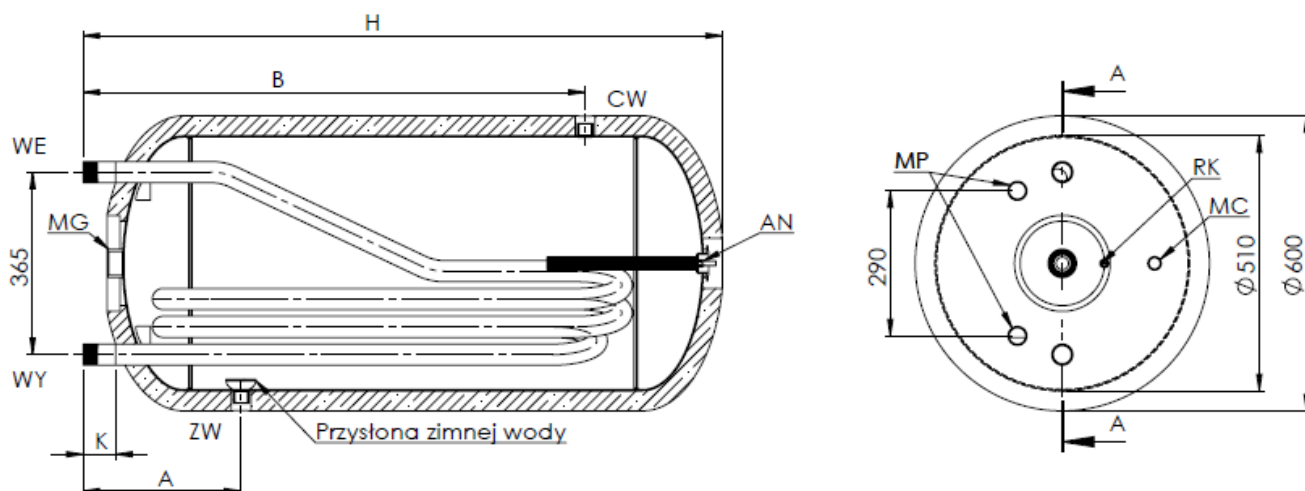
PRZEKRÓJ A-A
