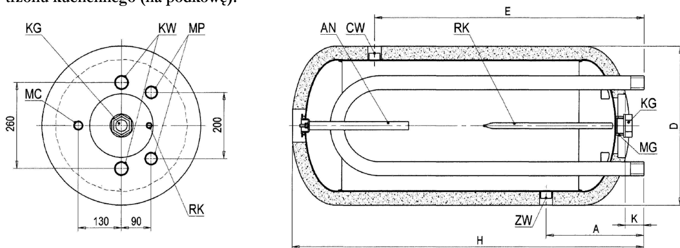
Rys.2b. Budowa i wymiary wymienników WGJ-g 140 z pojedynczą węzownicą z przyłączem do trzonu kuchennego (na podkowę).
