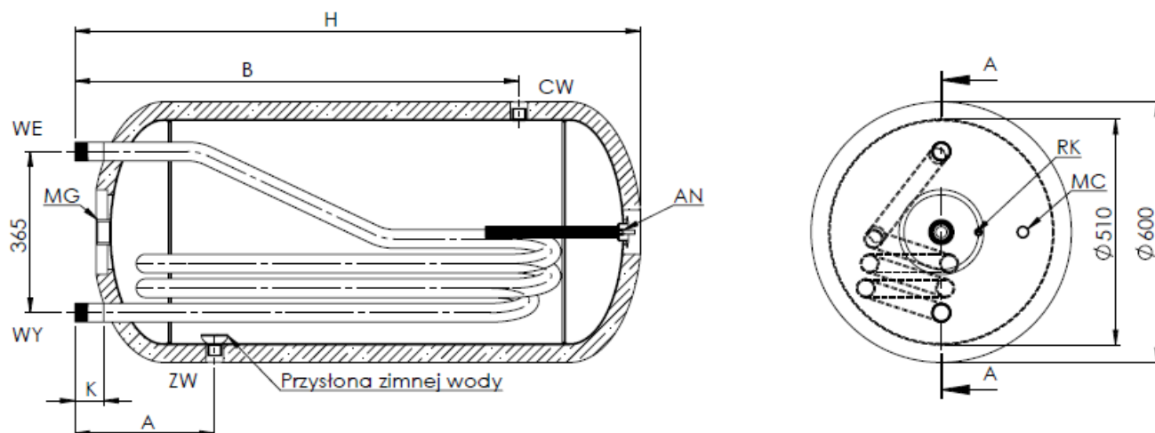
PRZEKRÓJ A-A
