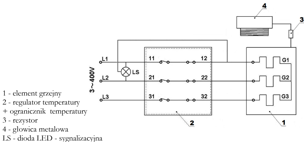
Rys. 3 Schemat instalacji elektrycznej
