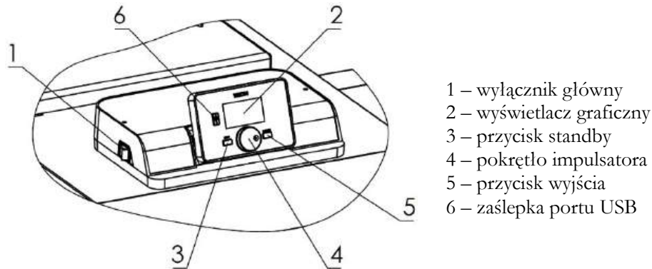
Rys. 3a. Panel sterujący sterownika EL-683 zPID
