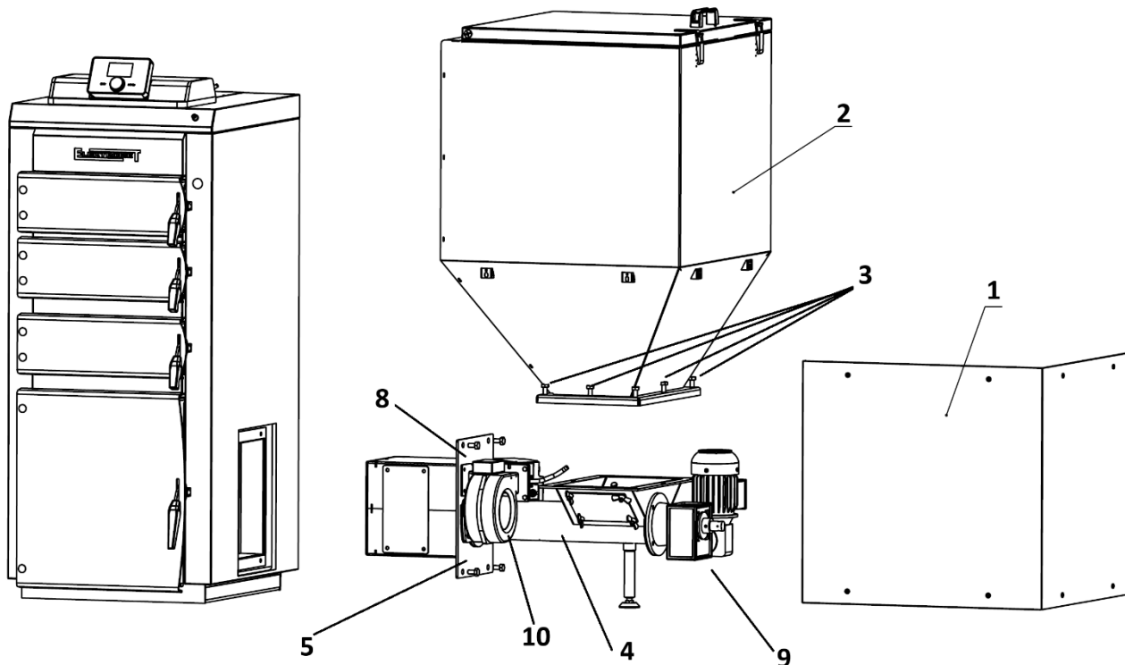
Rys. 5a. Elementy składowe układu palnika wraz z zasobnikiem.
