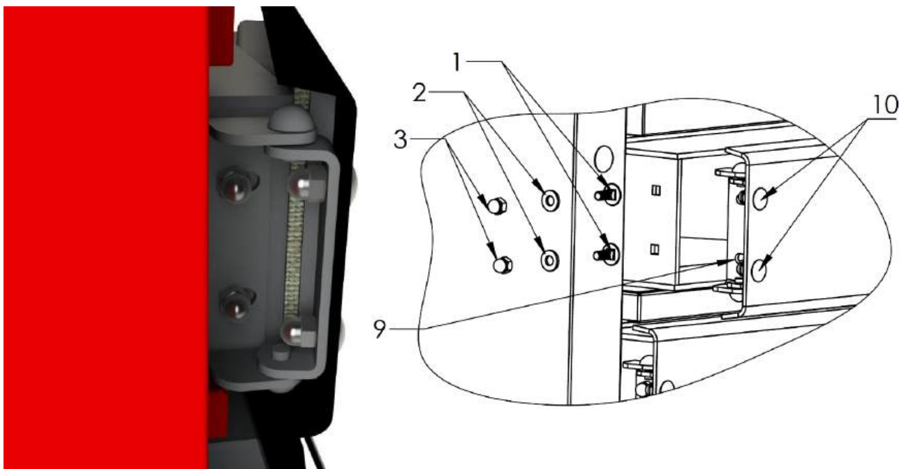
Rys.6b. Zawias drzwiczek
