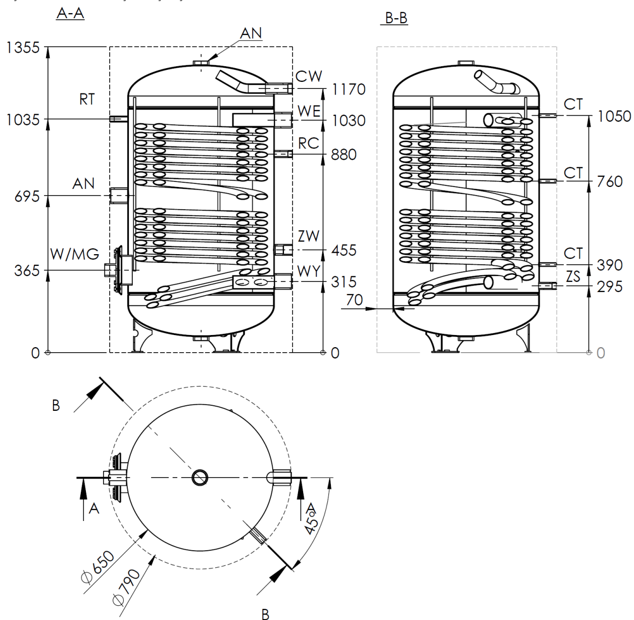
Rys. 1. Budowa i wymiary wymienników MEGA MAX 300.
