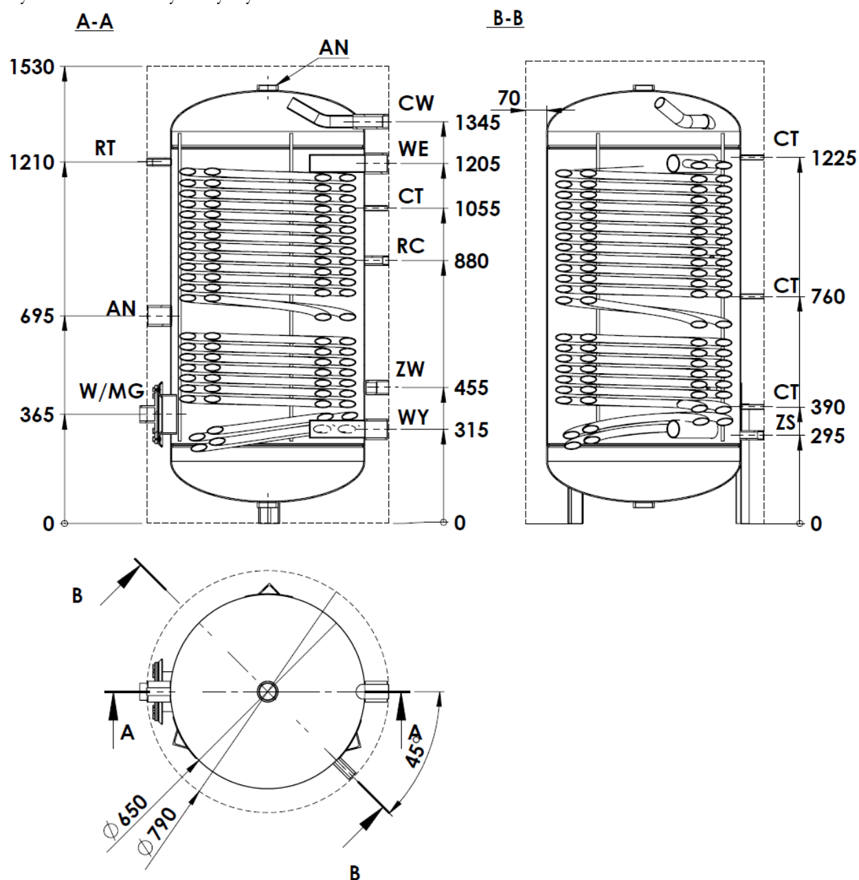
Rys. 2. Budowa i wymiary wymienników MEGA MAX 400.
