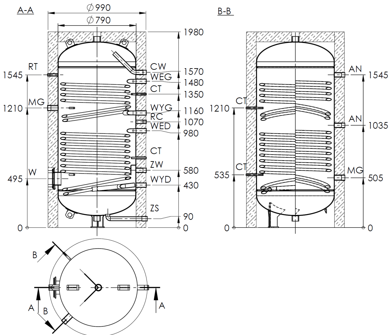
Rys.1 Budowa podgrzewacza WGJ- S 750 DUO
