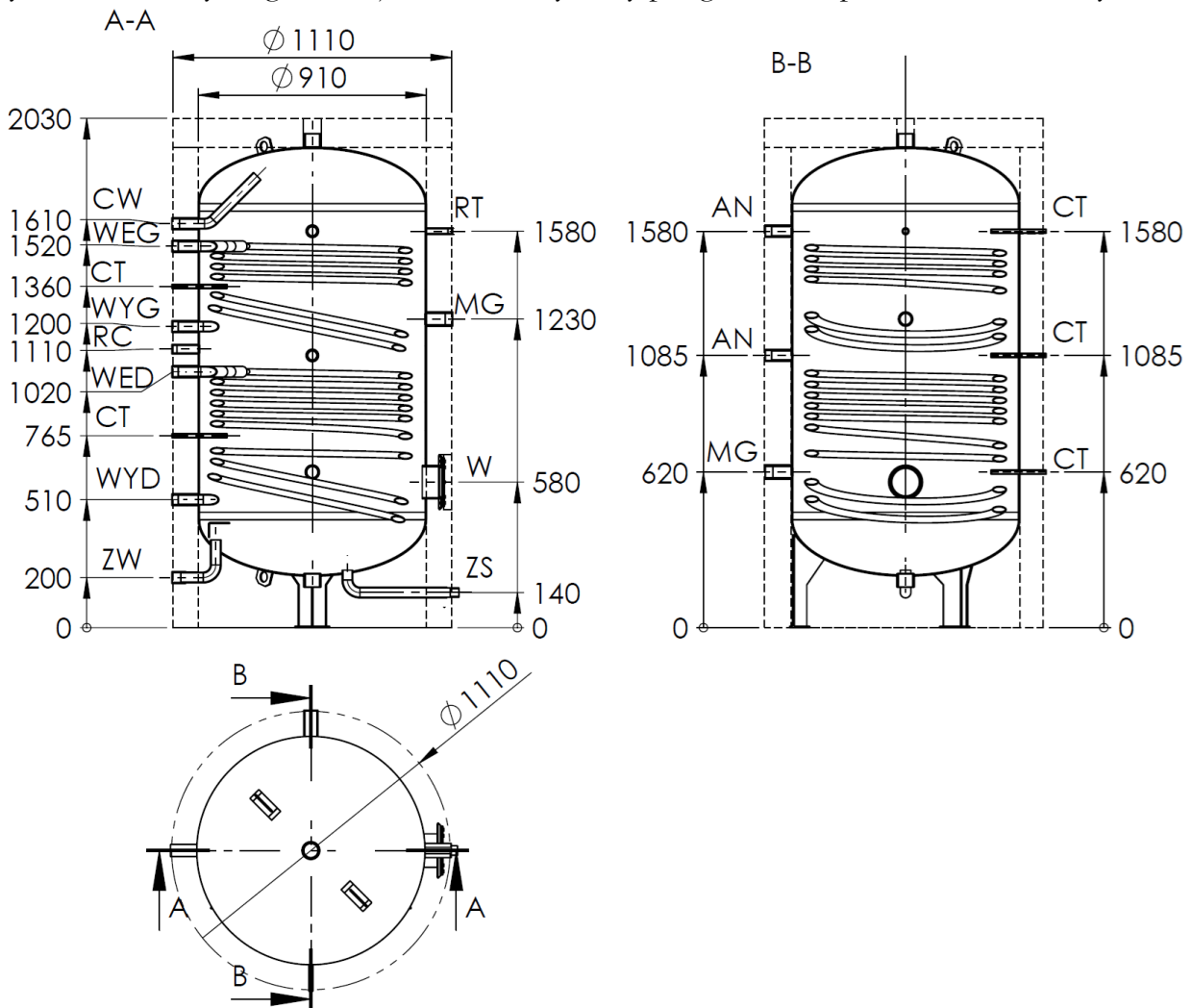
Rys.1 Budowa podgrzewacza WGJ- S 1000 DUO
