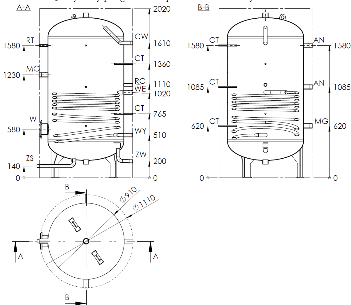
Rys.1 Budowa podgrzewacza WGJ- S 1000/2,8
