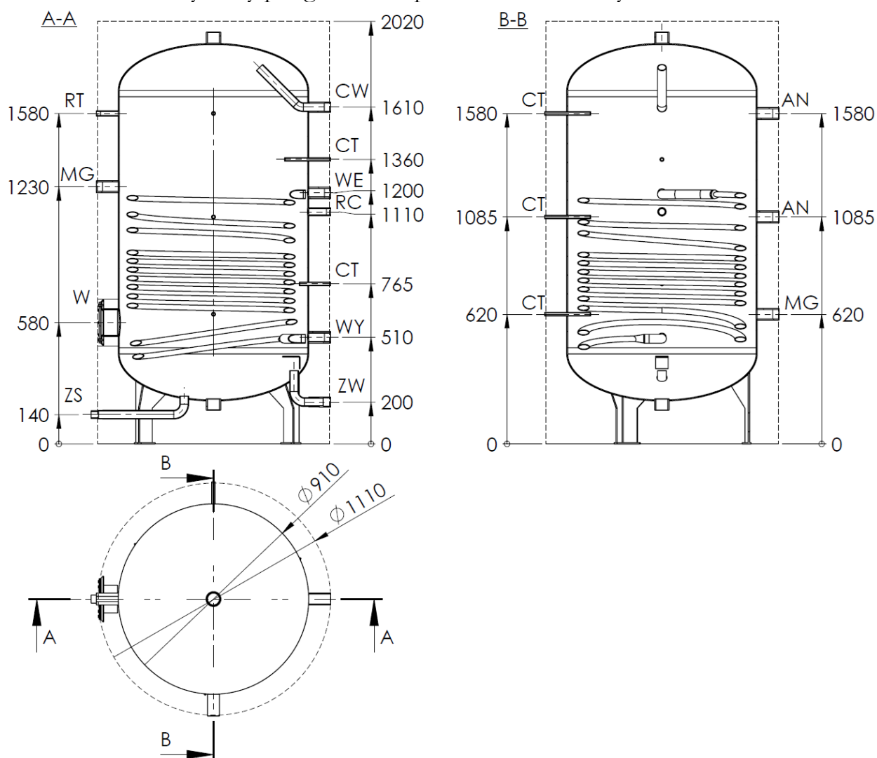
Rys.1 Budowa podgrzewacza WGJ- S 1000/3,7
