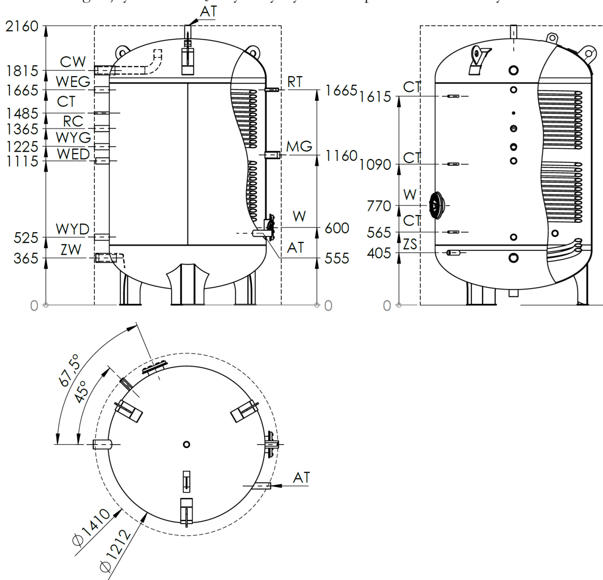
Rys.1 Budowa wymiennika WDP2 2000
